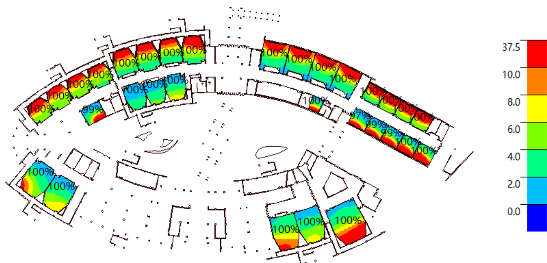
图 10 一层照度彩图
