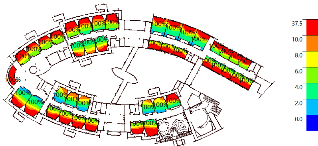
图 12 四层照度彩图
