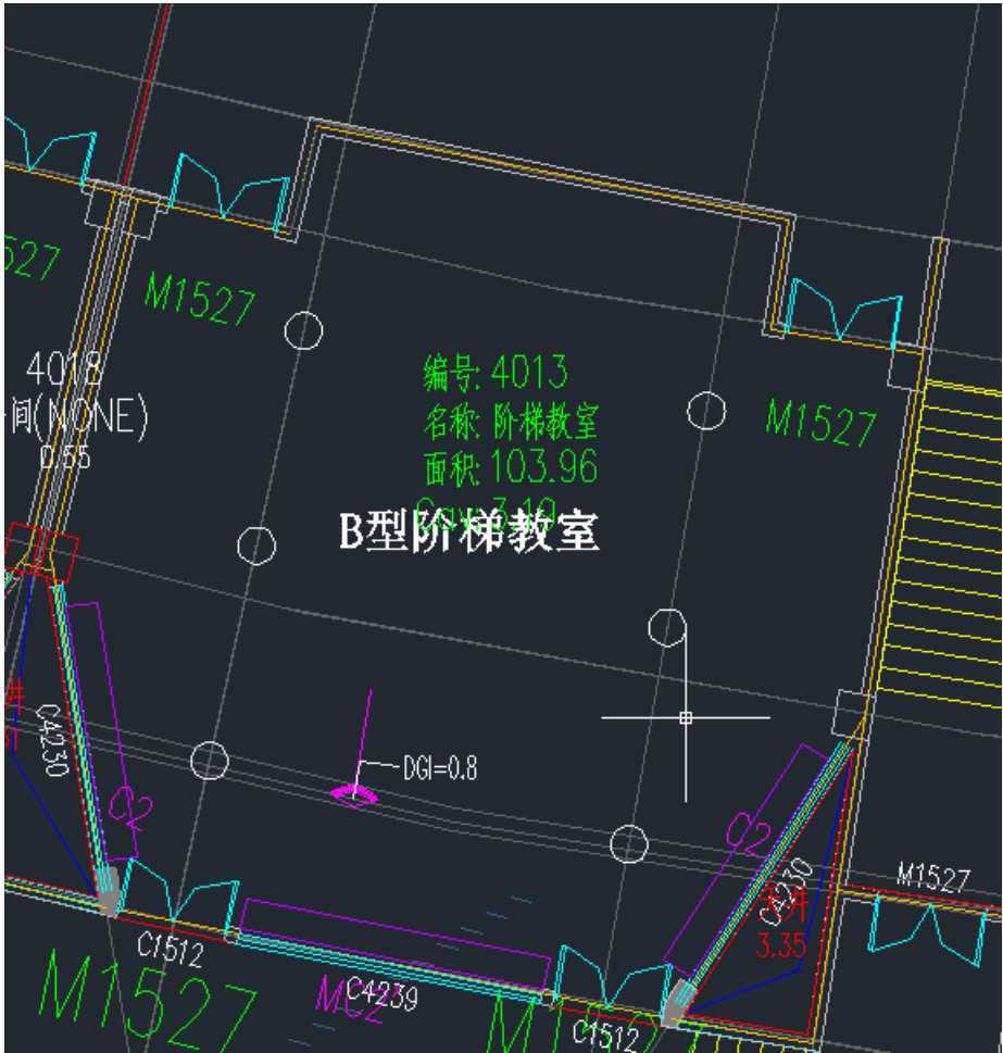
图 5 导光管+反光板教室布置
