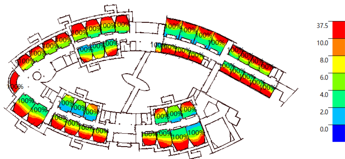
图 11 三层照度彩图
