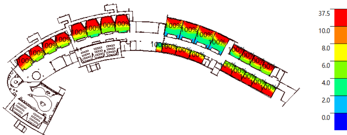
图 12 四层照度彩图
