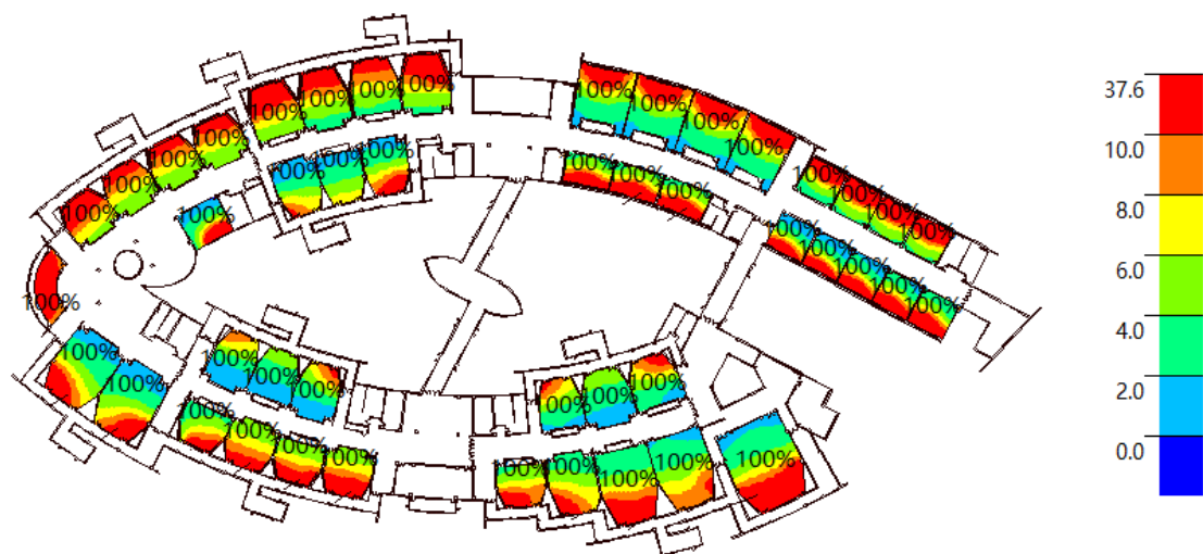
图 10 二层照度彩图
