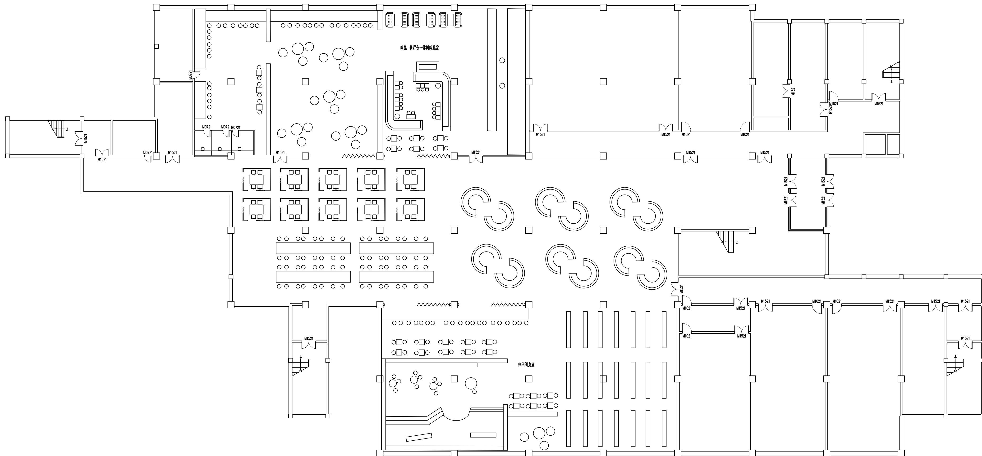
地下一层平面图 1:100
