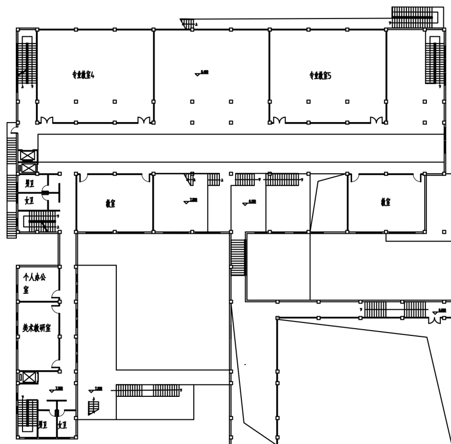
三层平面图1: 500
