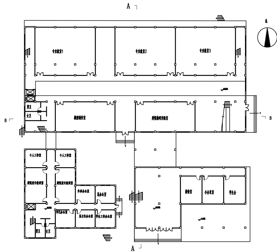
一层平面图1: 500
