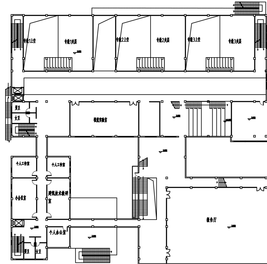
二层平面图1: 500
