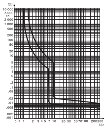
图1 C型热/电磁脱扣特性曲线
