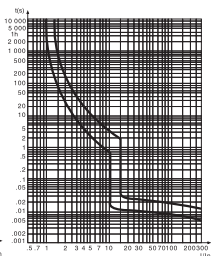
图2 D型热/电磁脱扣特性曲线
