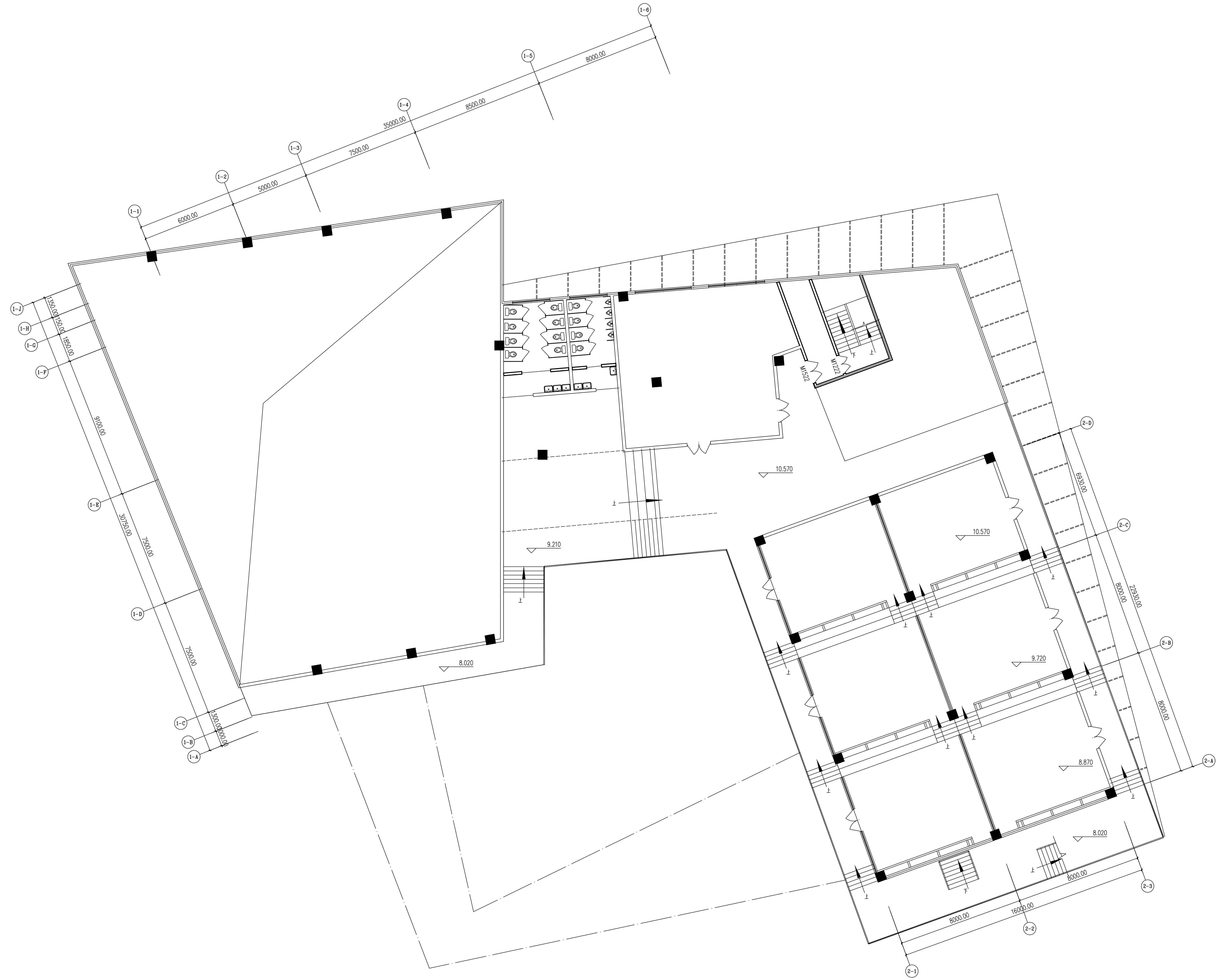
三层平面 1:100
