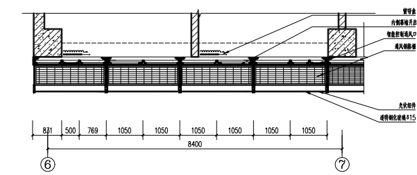
A-A 双层幕墙横剖大样图 1:50
