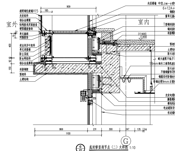
2 JD 出风口竖剖节点大样图 1:10
