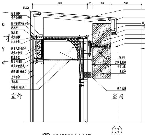
7 JD 顶封竖剖节点(一)大样图 1:10
