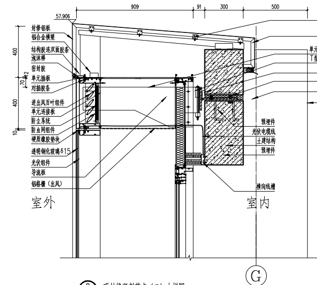
8 JD 顶封竖剖节点(二)大样图 1:10
