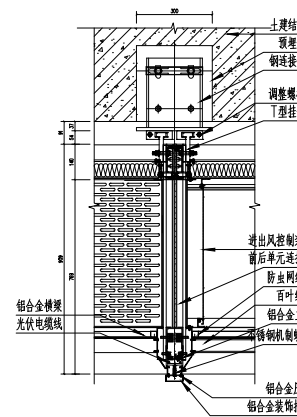
4 JD 通风口处横剖节点大样图 1:10
