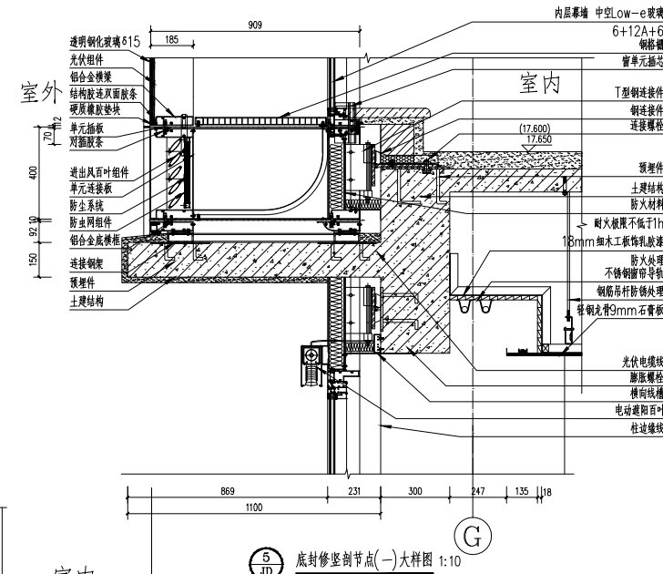
1 JD 进风口竖剖节点大样图 1:10
