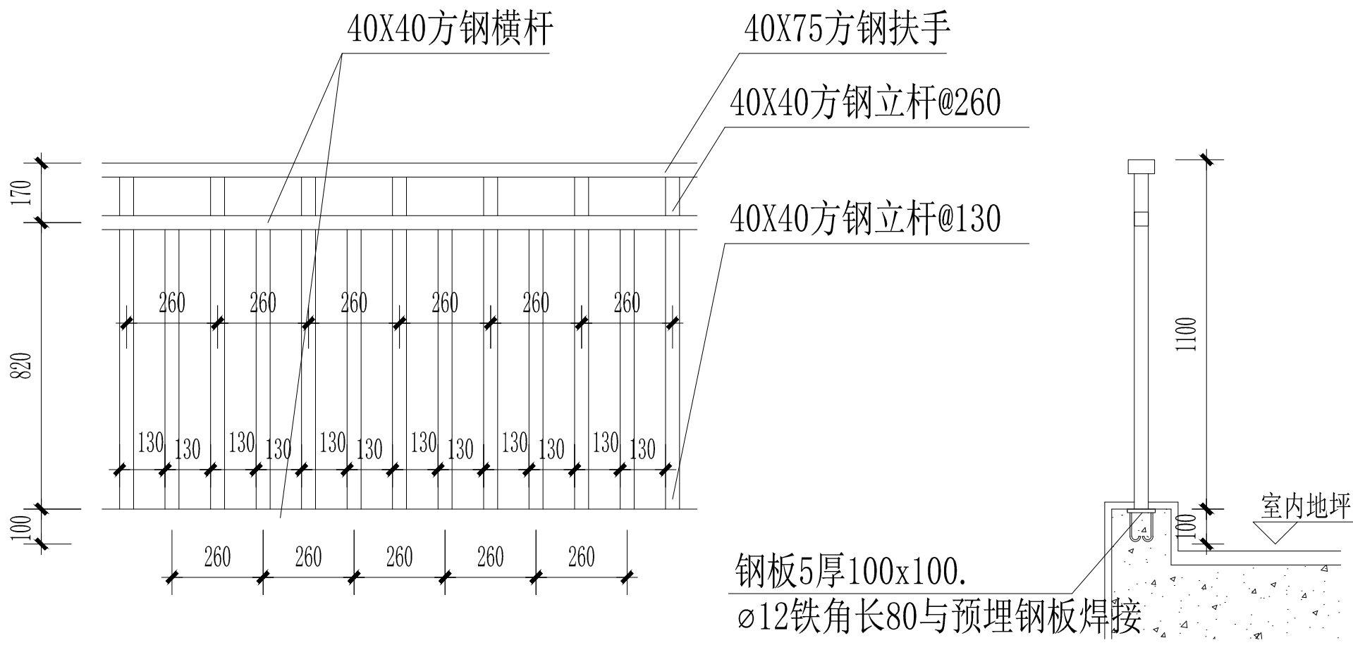
阳台栏杆详图 (一) 1:20
