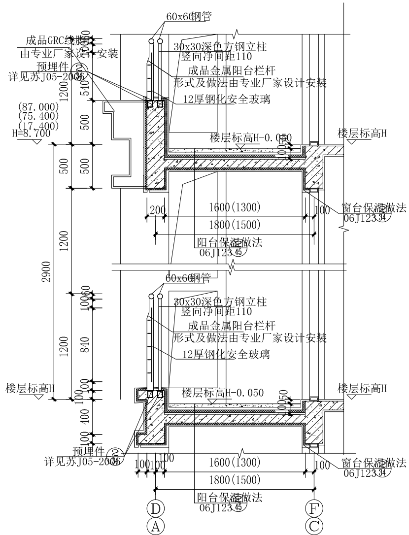
阳台1 1-1剖面 1:25
