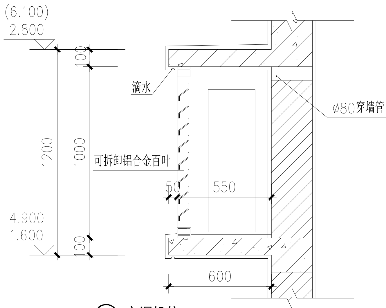
空调机位 1:20
