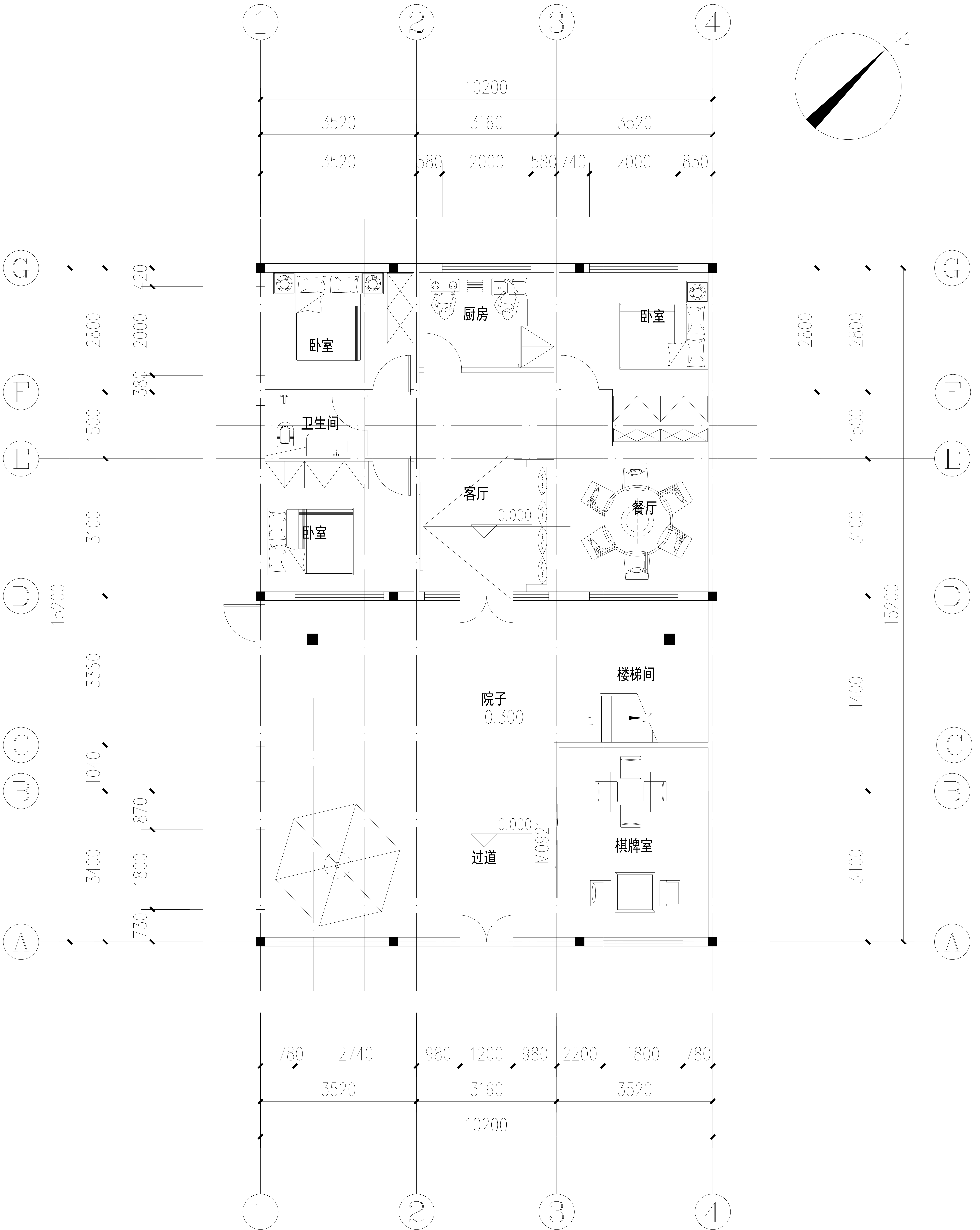
一层平面图 1:100
