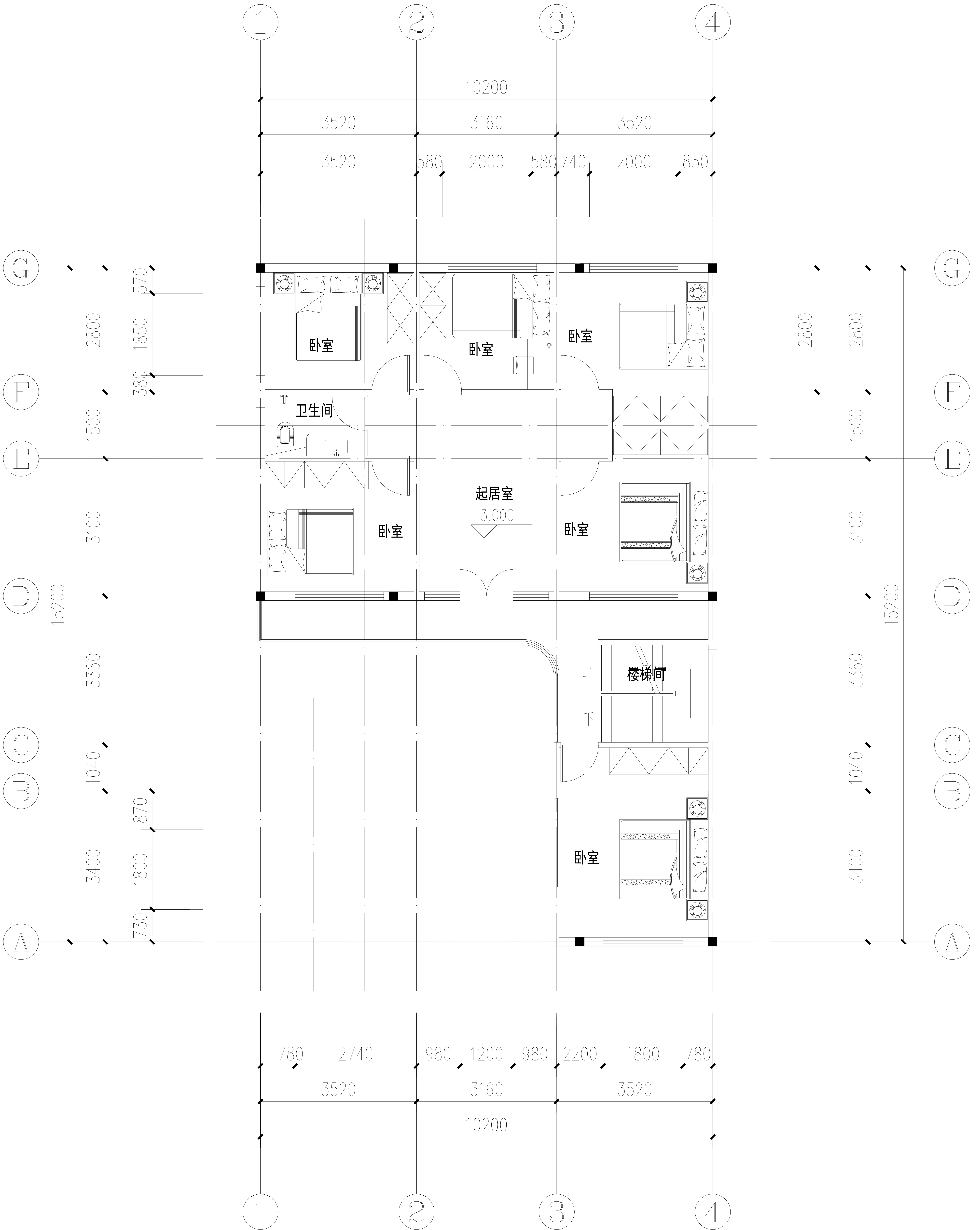
二层平面图 1:100
