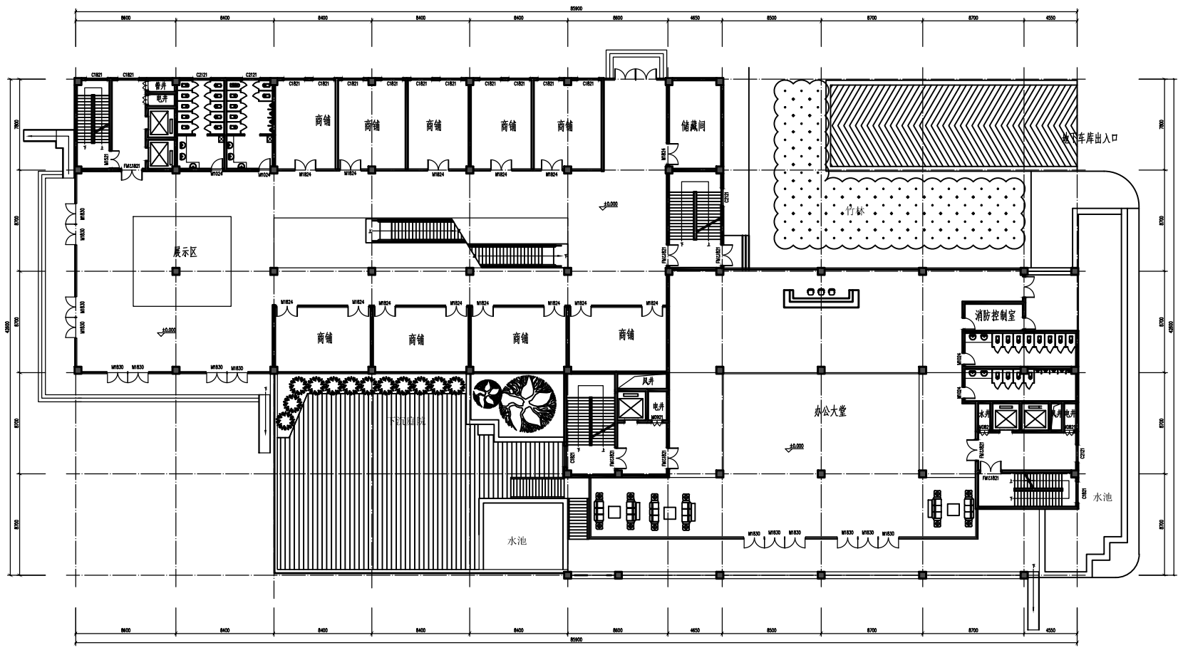
一层平面图 1:100
