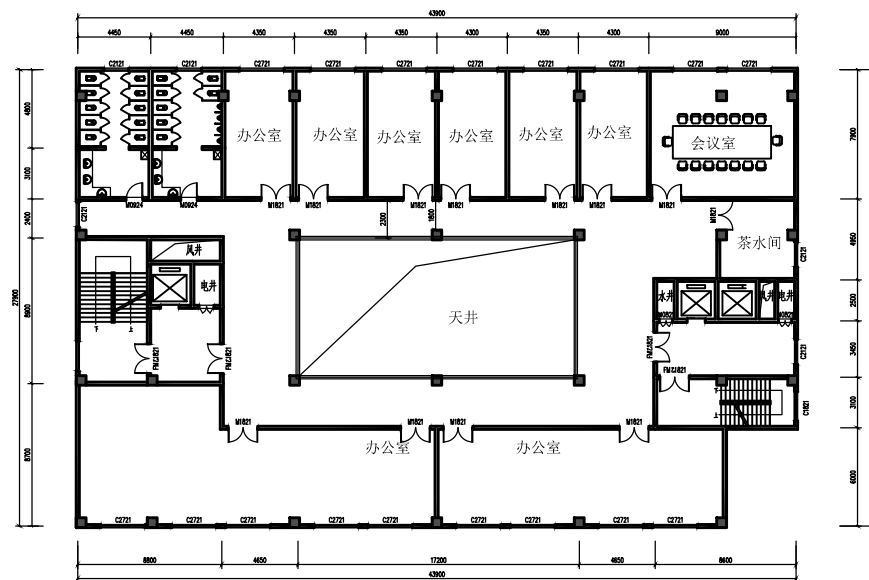
四~十层平面图 1:100
