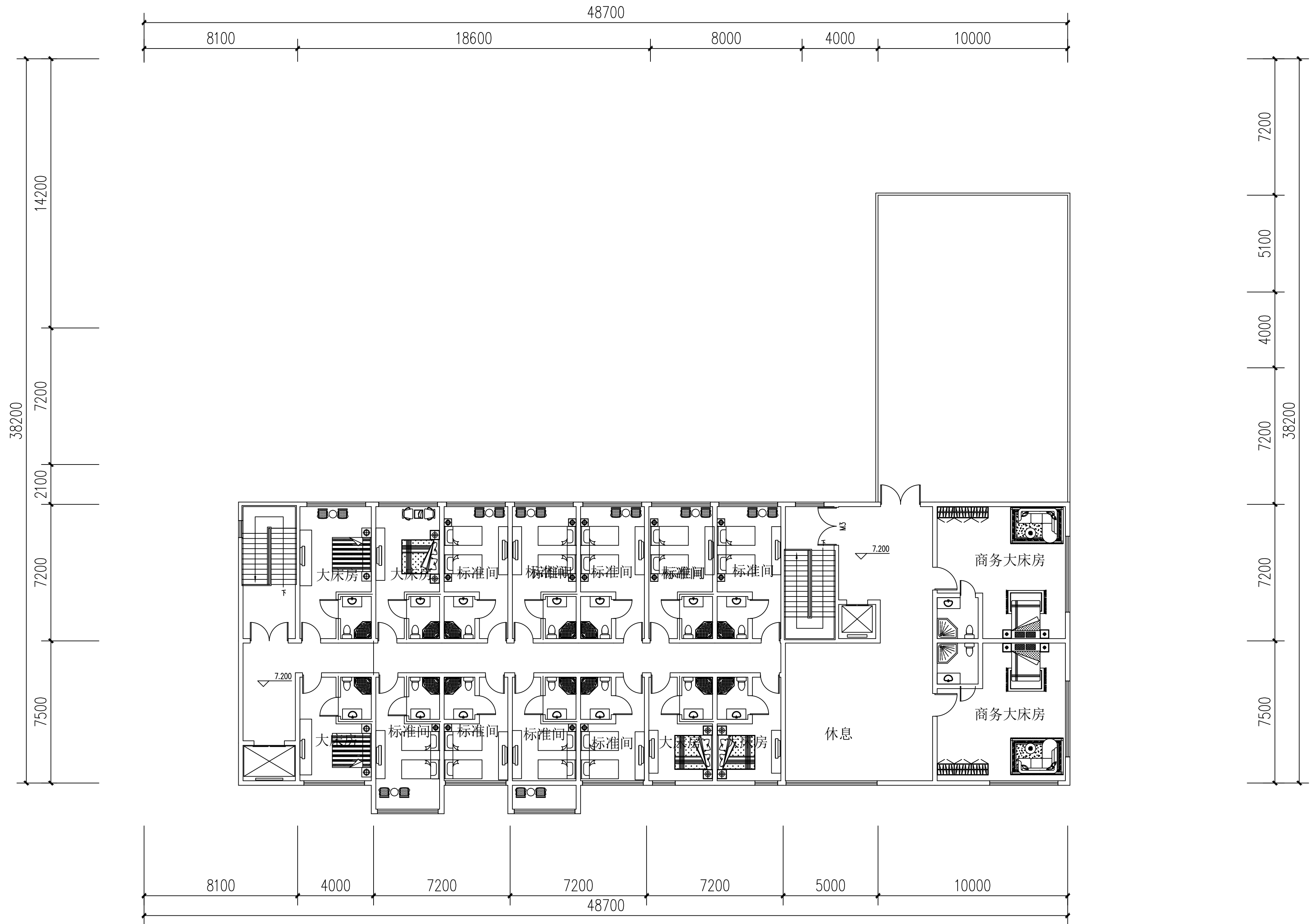
三层平面图 1:100
