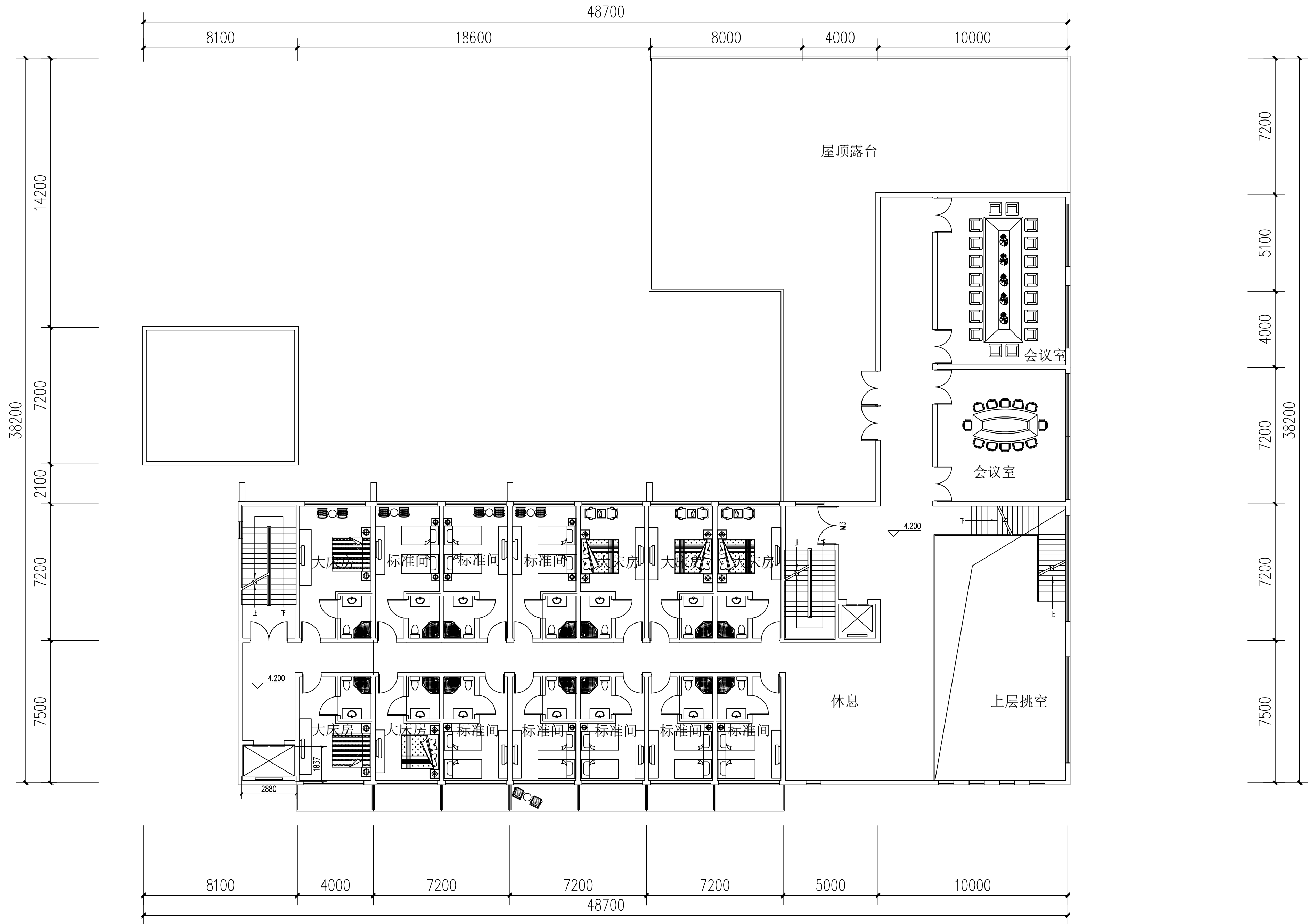
二层平面图 1:100
