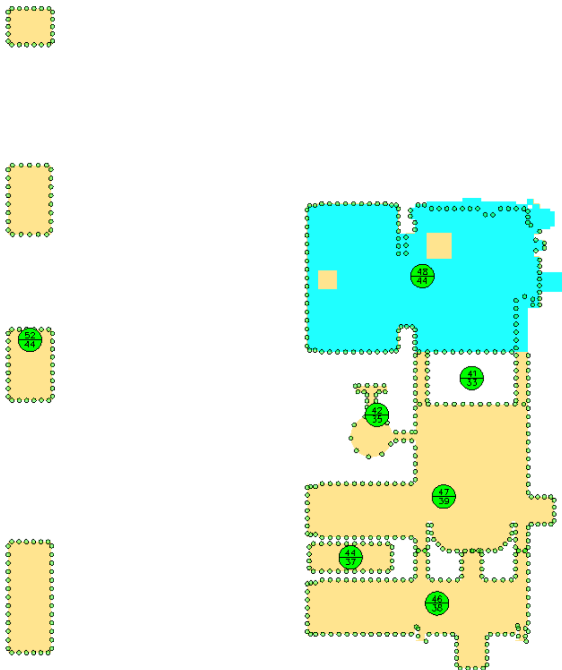
图 4.2-1 参评建筑附近区域 1.5m 高度处声压级平面分布图（昼间）
