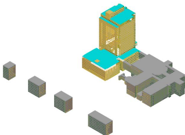
图 4.2-3 参评建筑附近区域声压级鸟瞰分布图（昼间）
