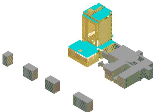
图 4.2-4 参评建筑附近区域声压级鸟瞰分布图（夜间）
