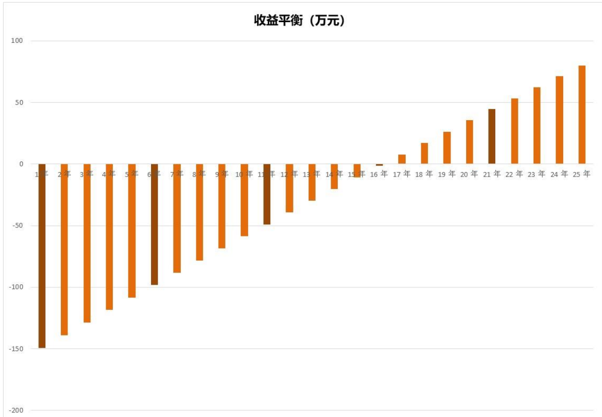
图 13 收益平衡图
