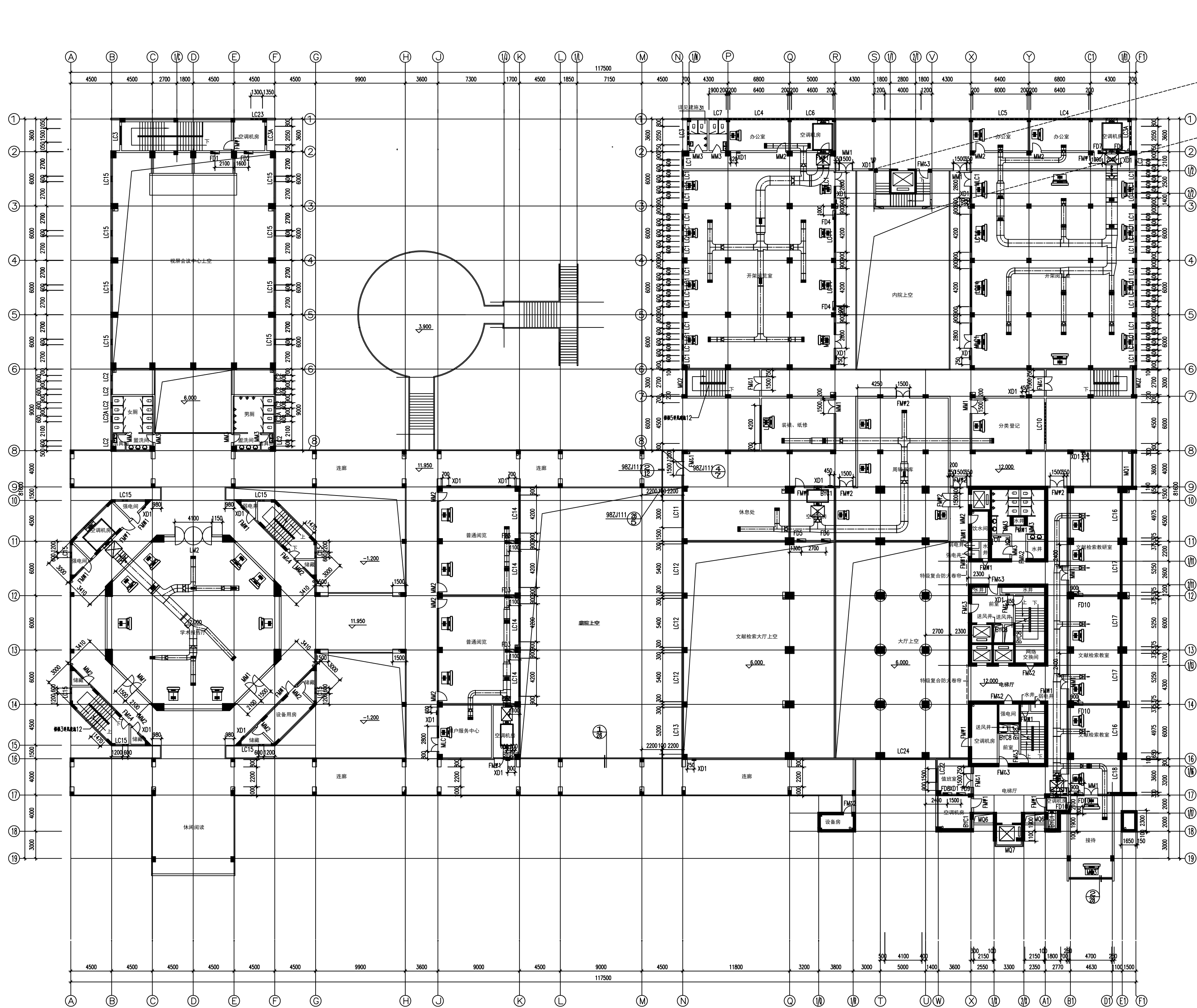
三层平面图 1:150
