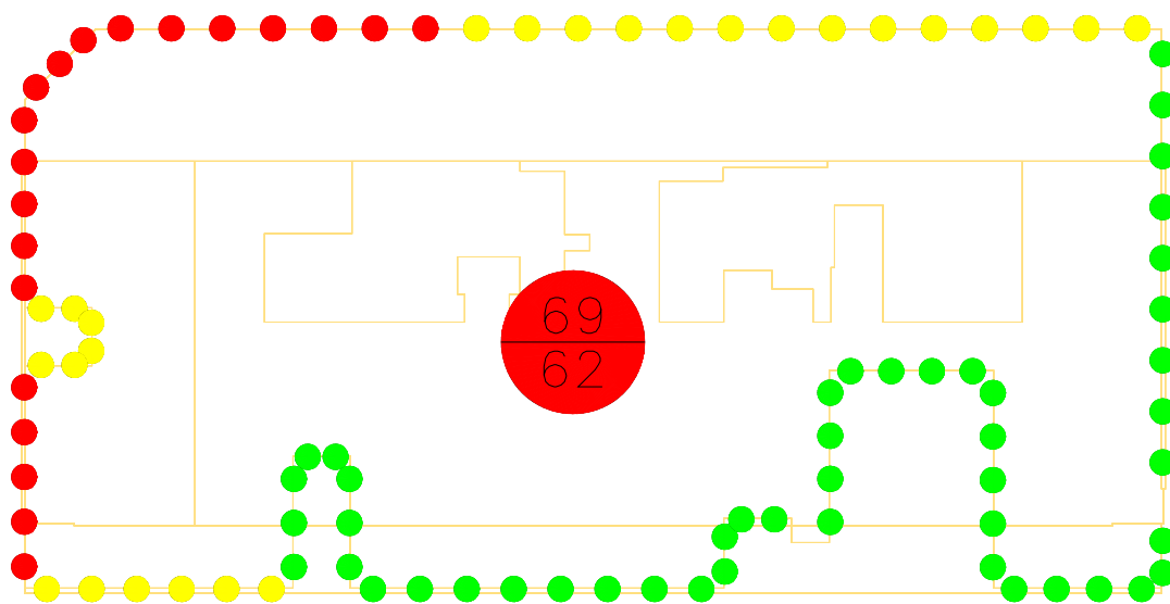
图 4.2-1 参评建筑附近区域 1.5m 高度处声压级平面分布图（昼间）
