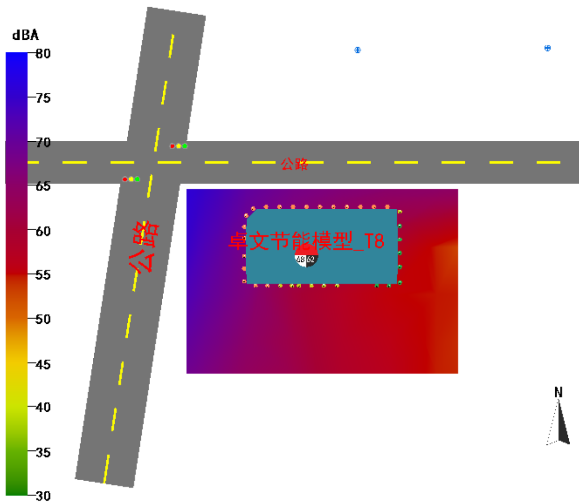
图 4.1-1 场地 1.5m 高度处声压级分布图 (昼间)
