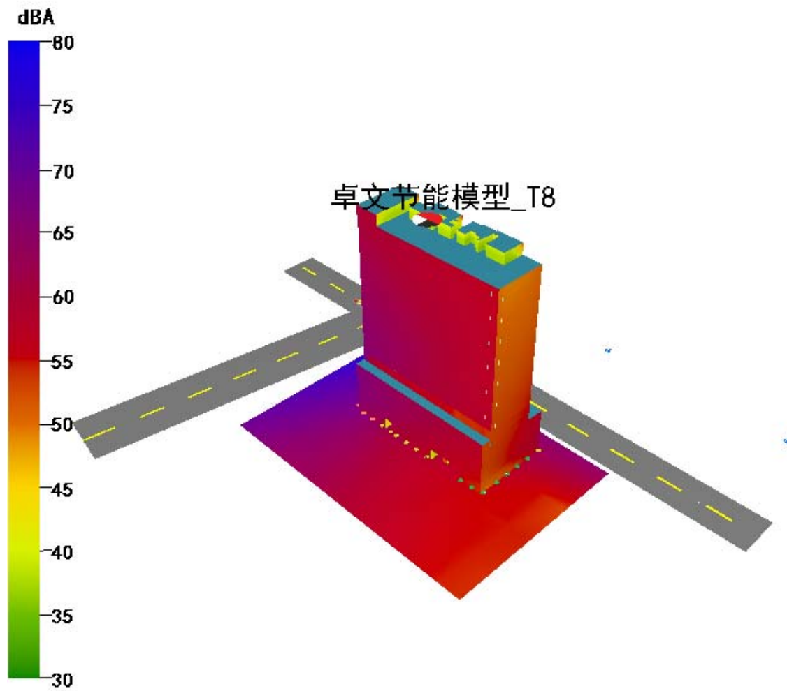
图 4.1-3 场地噪声分布俯瞰图（昼间）
