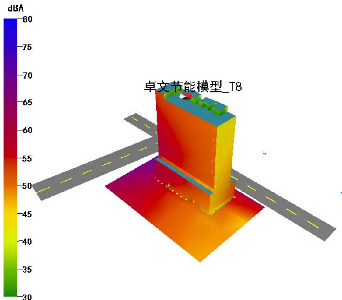
图 4.1-4 场地噪声分布俯瞰图（夜间）
