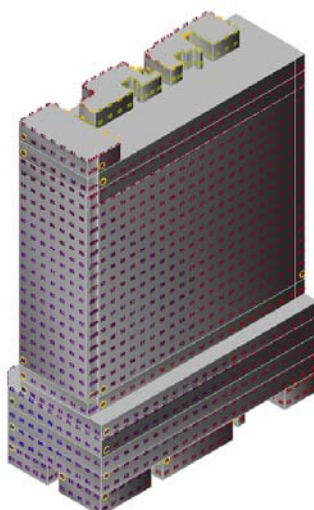
图 4.2-4 参评建筑附近区域声压级鸟瞰分布图（夜间）
