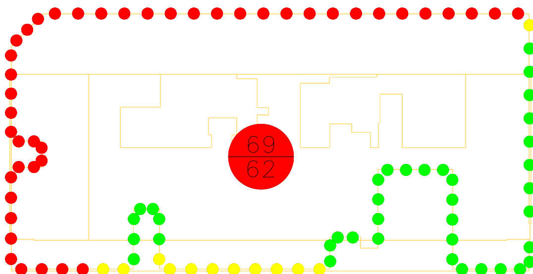
图 4.2-2 参评建筑附近区域 1.5m 高度处声压级平面分布图（夜间）
