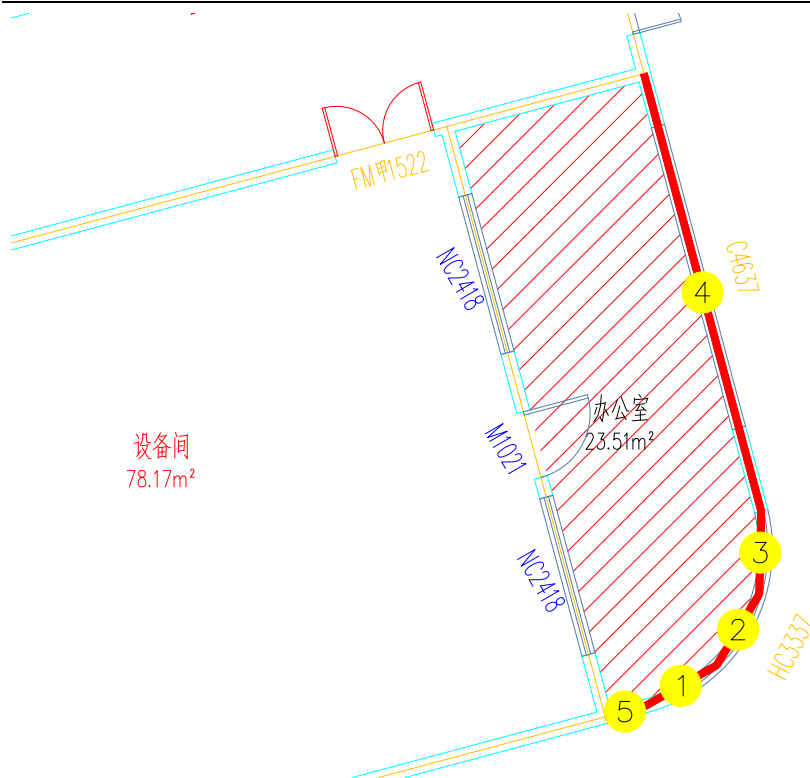
图 5-2 房间围护结构示意图
