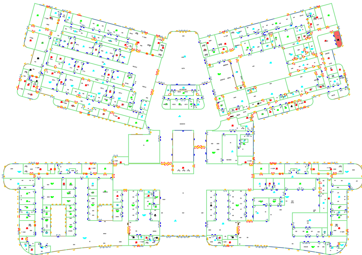
图 5-1 典型房间楼层平面图
