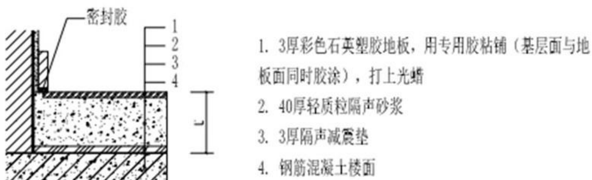
图 6.5 手术室(分娩室)与上层房间之间楼板
