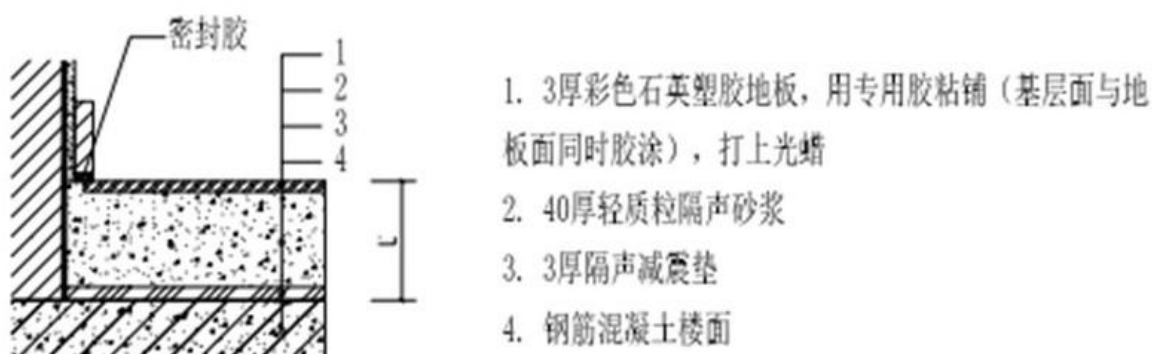
图 6.6 病房与上层房间之间楼板
