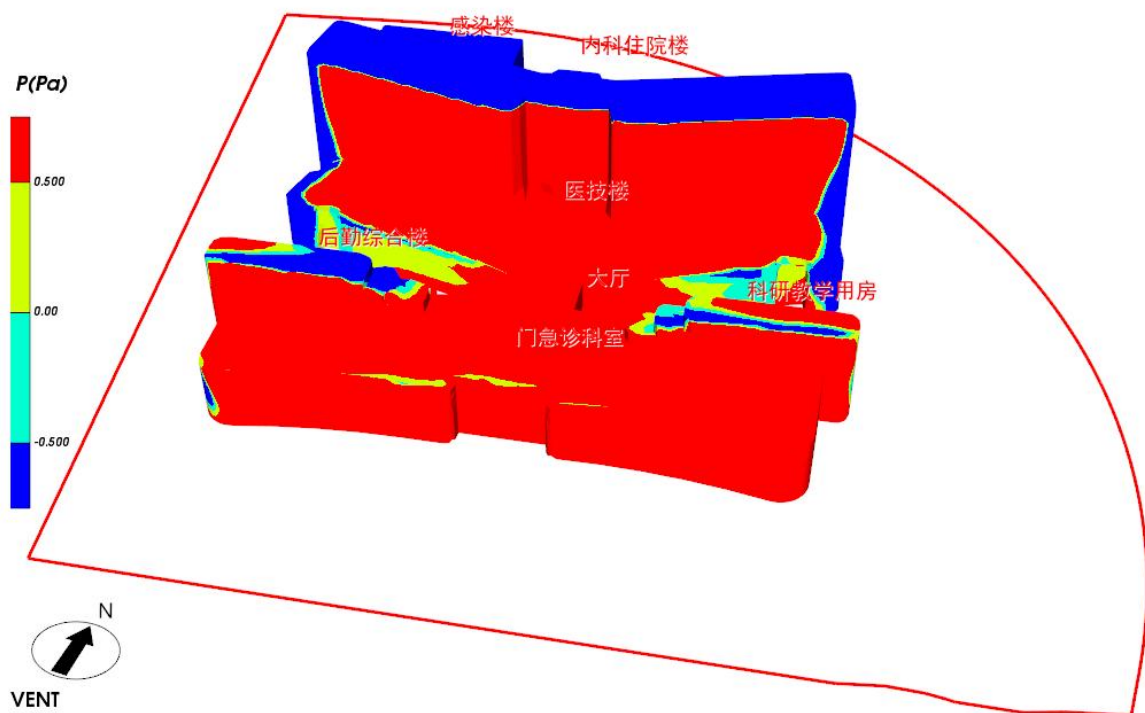
图 5.3- 1 建筑迎风面外窗表面风压云图-夏季
