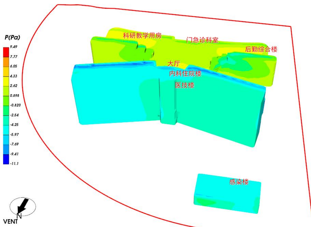
图 5.2- 5 建筑背风面风压云图
