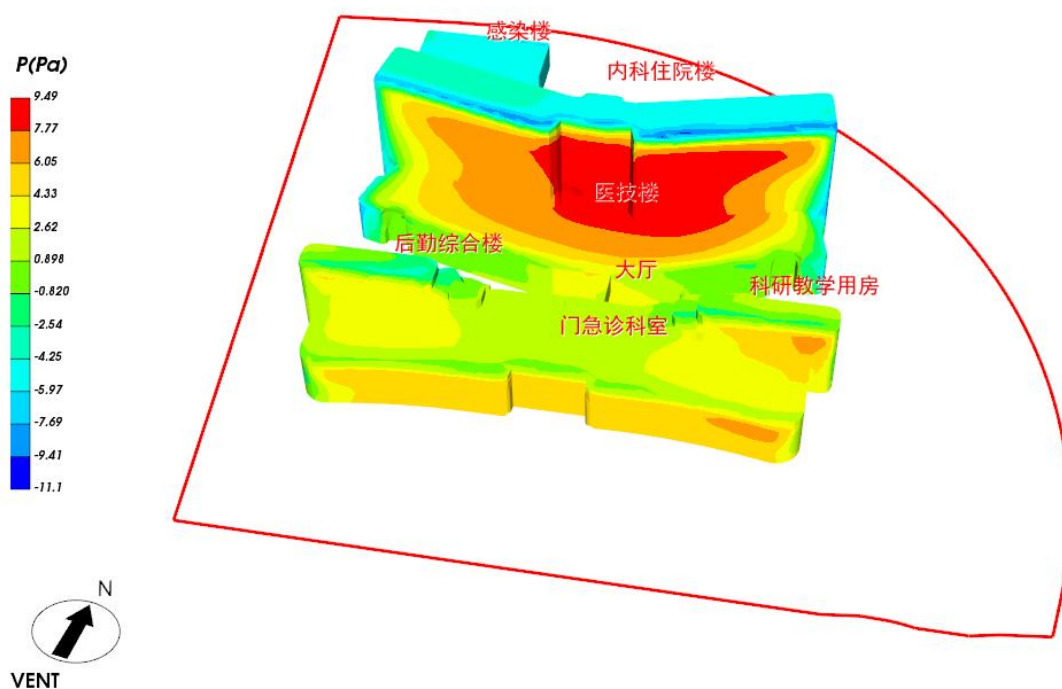
图 5.2- 4 建筑迎风面风压云图
