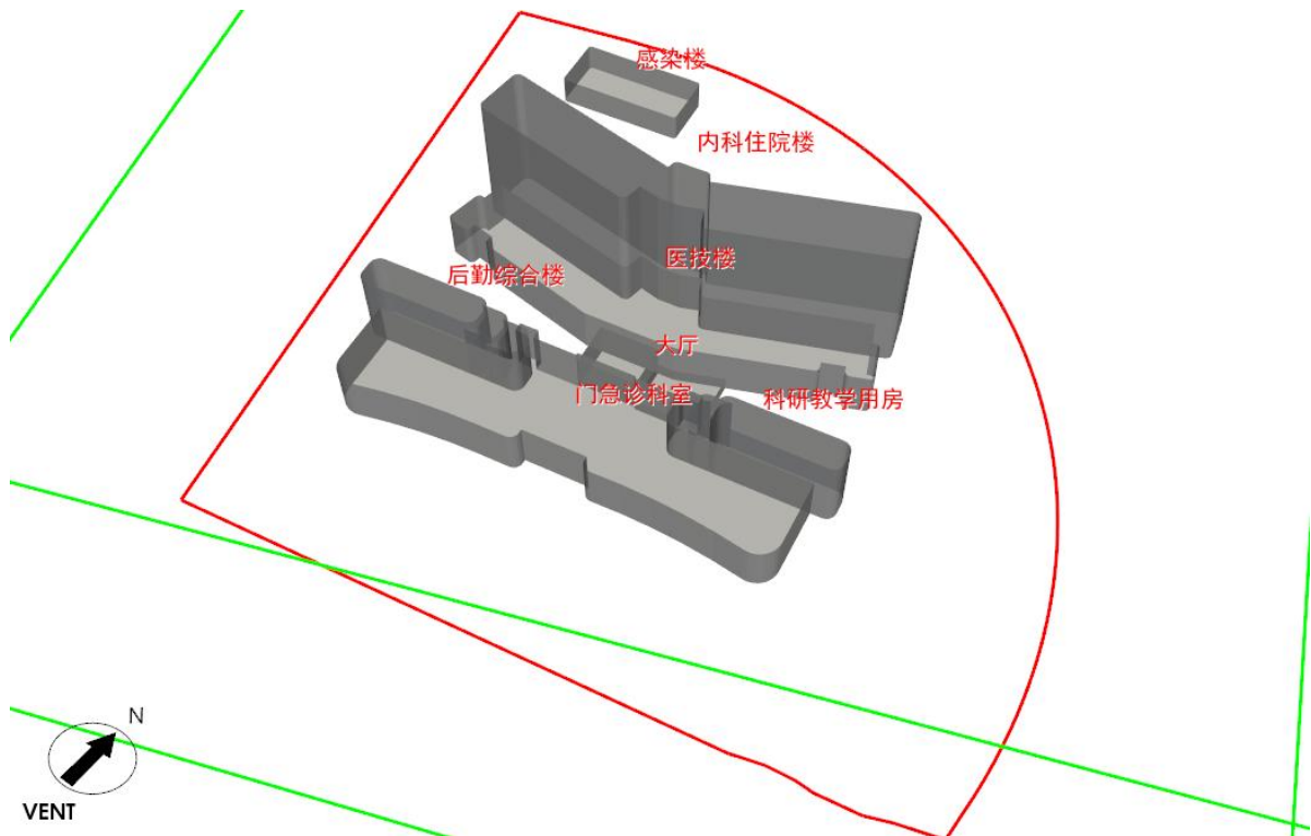
图 4.1-3 过渡季工况风场计算域图示
