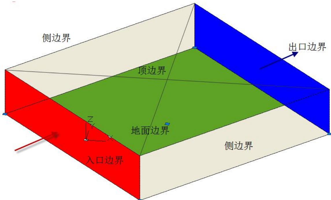
图 4.3- 1 风场边界类型示意图
