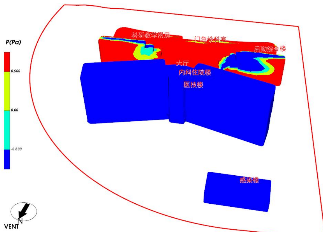
图 5.3- 2 建筑背风面外窗表面风压云图-夏季
