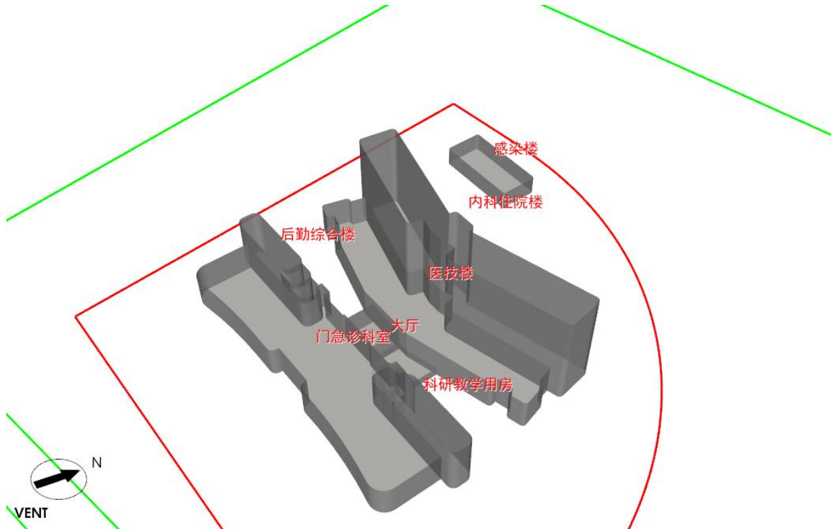
图 4.1-1 冬季工况风场计算域图示
