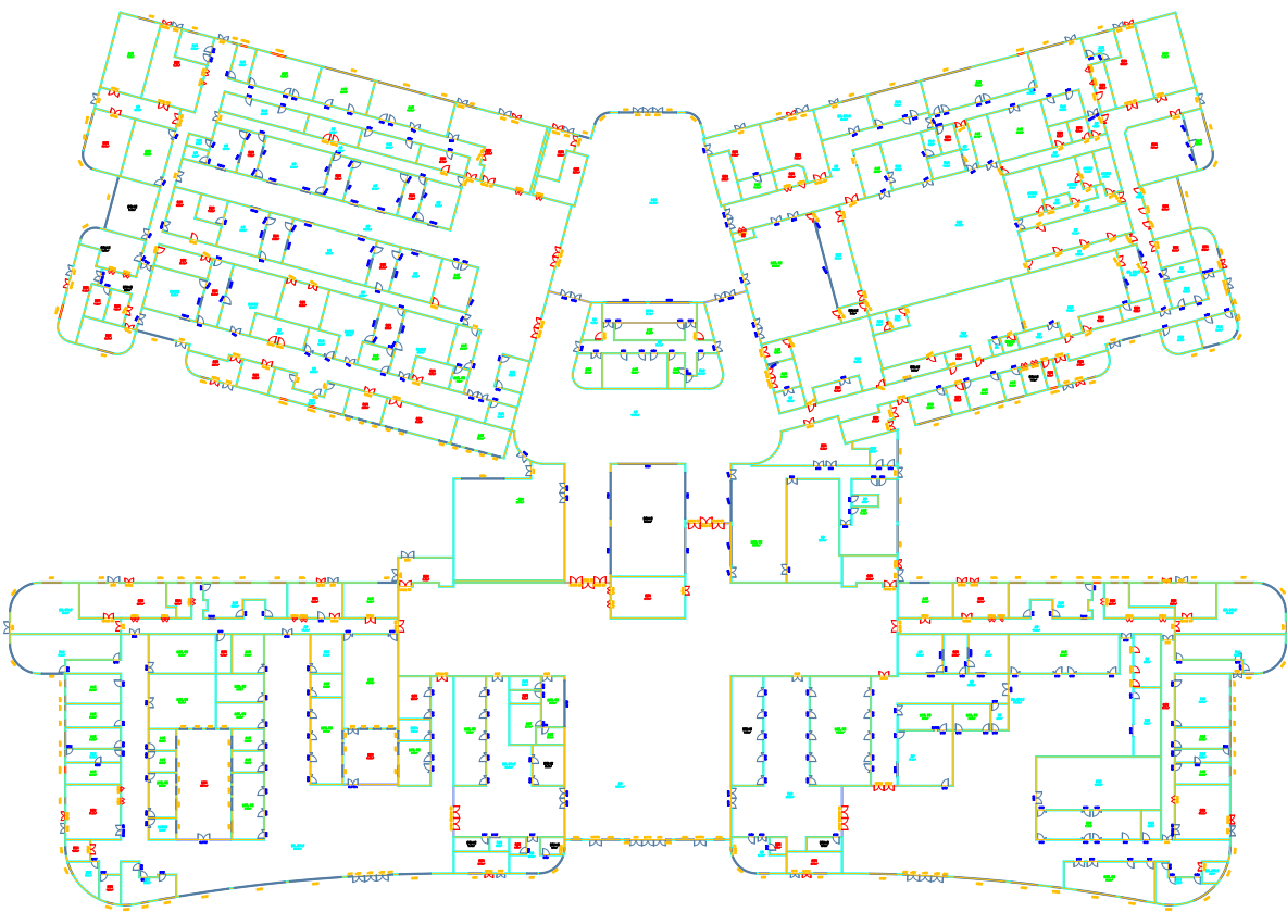
1 层平面
