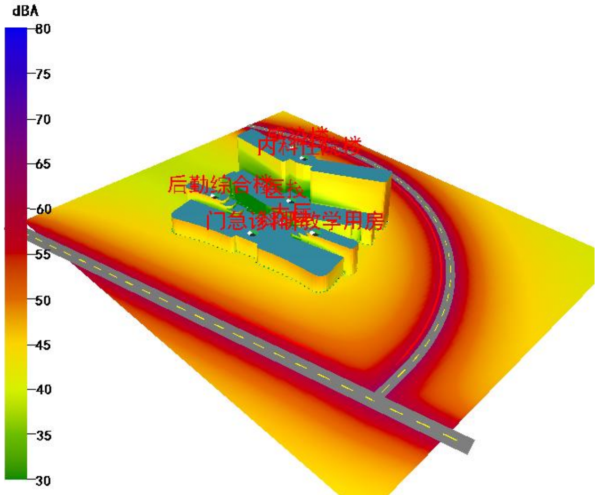
图 3.1-4 场地噪声分布俯瞰图（夜间）
