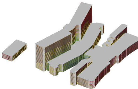
图 3.2-3 参评建筑附近区域声压级鸟瞰分布图（昼间）
