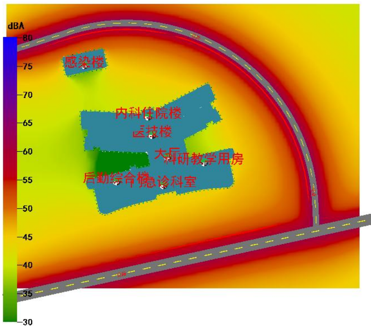
图 3.1-2 场地 1.5m 高度处声压级分布图（夜间）
