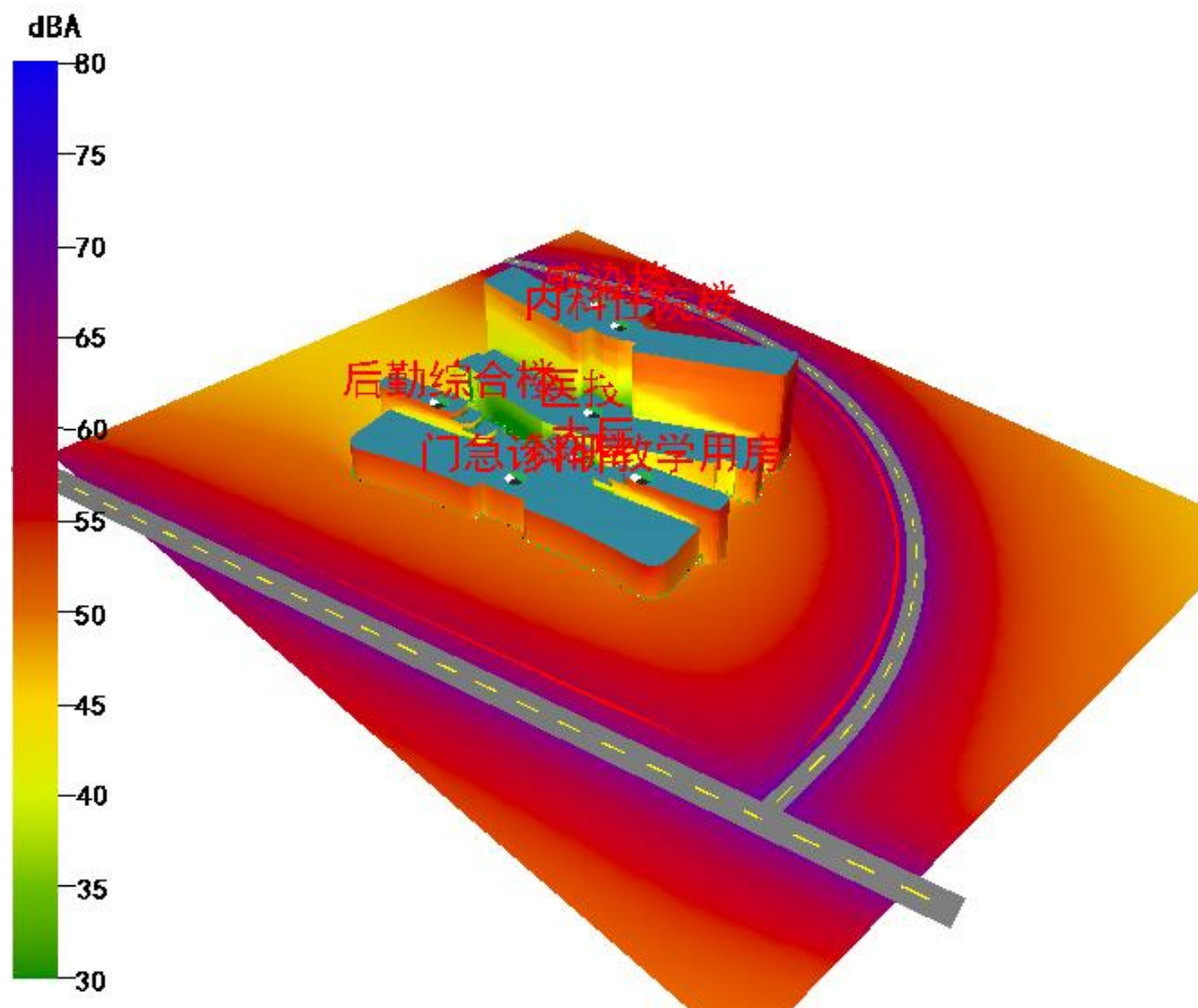
图 3.1-3 场地噪声分布俯瞰图（昼间）
