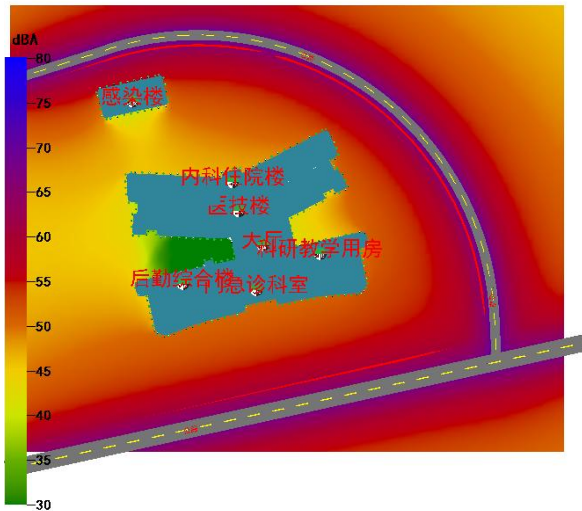
图 3.1-1 场地 1.5m 高度处声压级分布图 (昼间)
