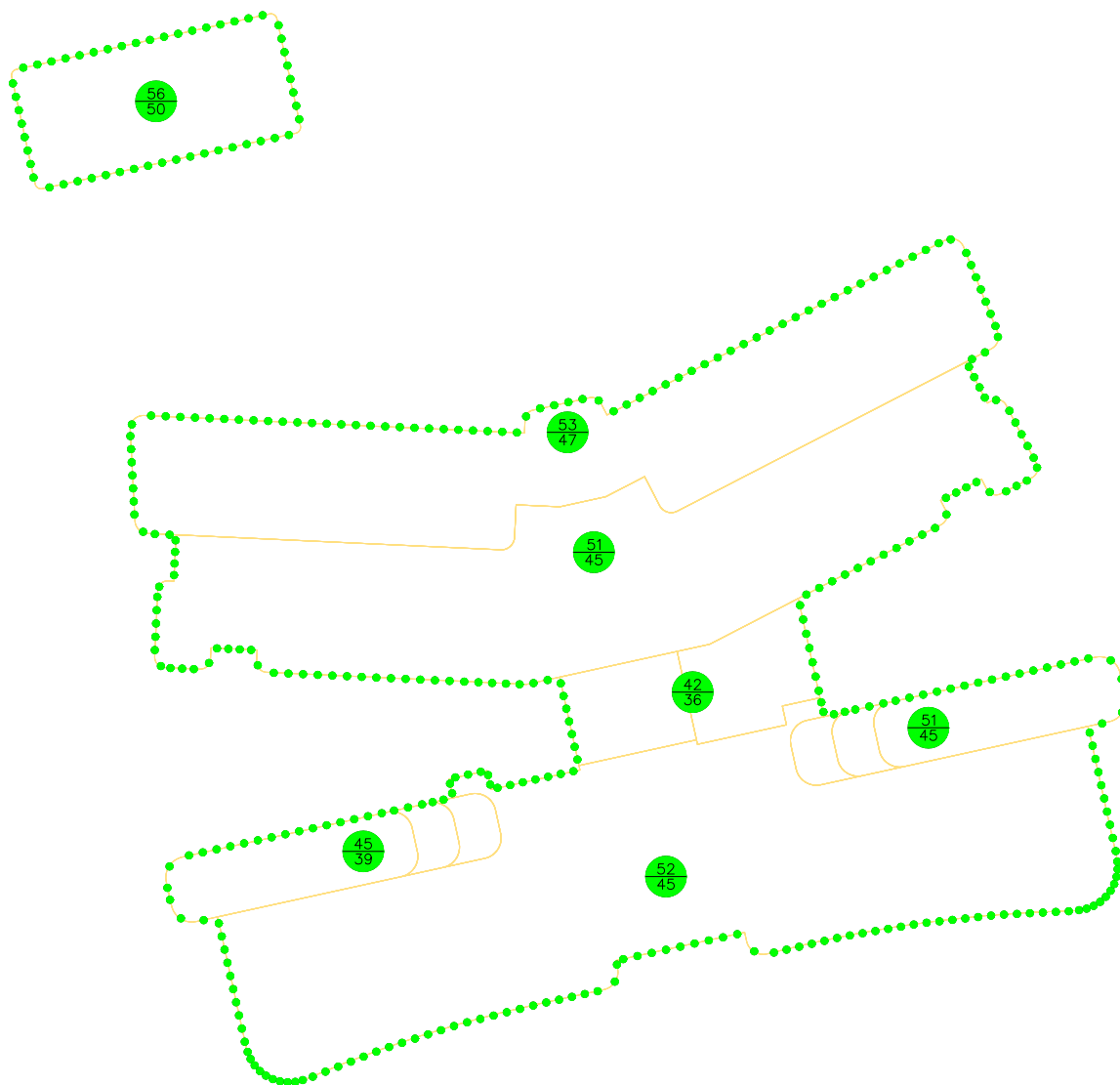
图 3.2-1 参评建筑附近区域 1.5m 高度处声压级平面分布图 (昼间)
