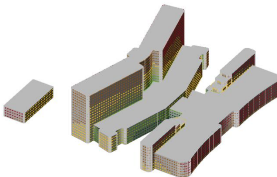
图 3.2-4 参评建筑附近区域声压级鸟瞰分布图（夜间）
