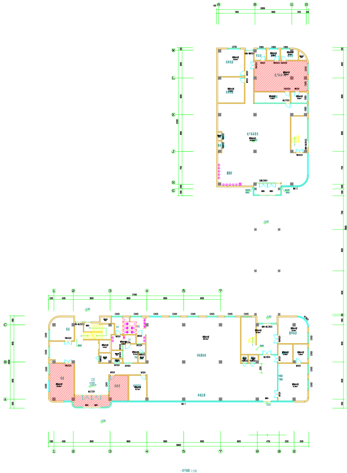
图 5- 1 受建筑外部噪声影响的典型房间楼层平面图
