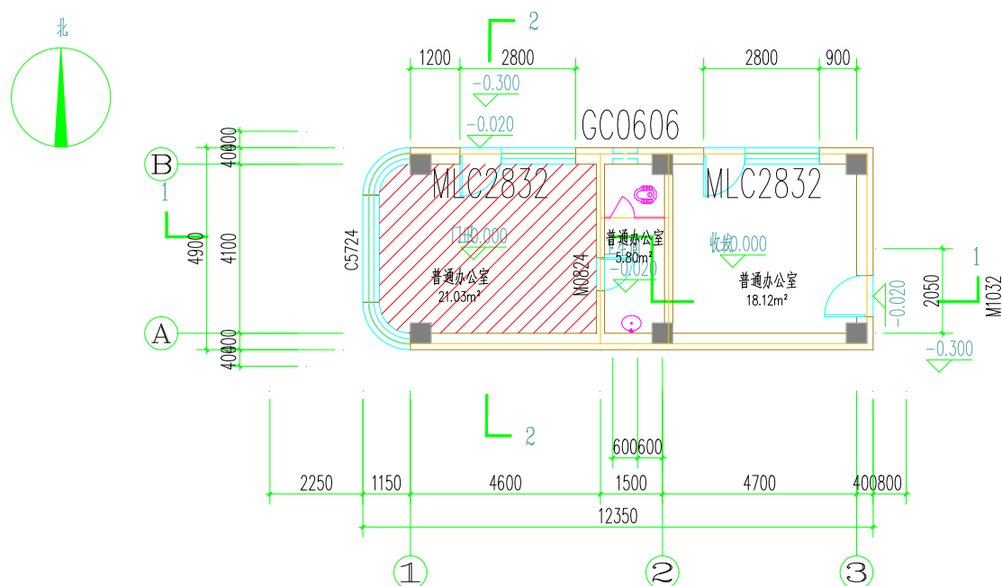
图 5-1 受建筑外部噪声影响的典型房间楼层平面图
