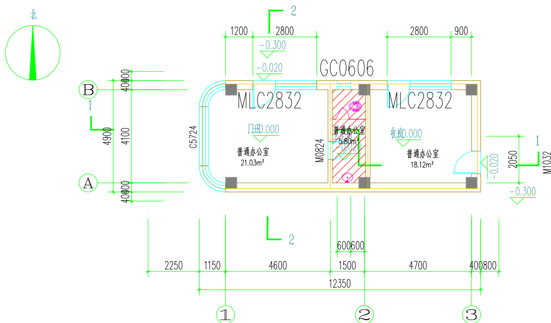
图 5-3 受建筑内设备噪声影响的典型房间楼层平面图
