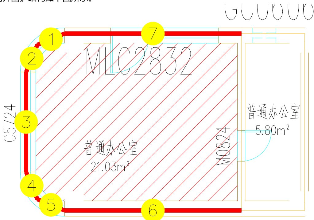
图 5- 2 典型房间外围护结构
