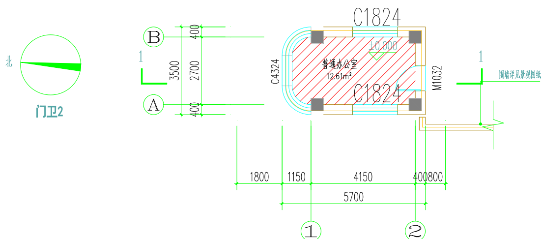
图 5-1 受建筑外部噪声影响的典型房间楼层平面图
