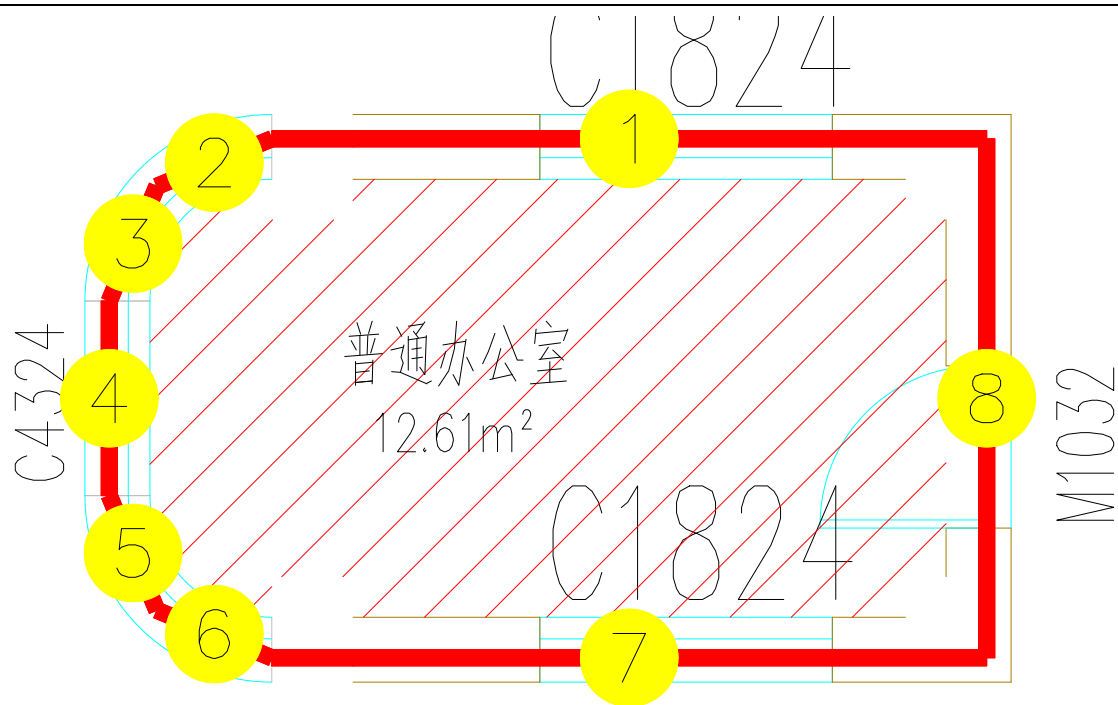
图 5- 2 典型房间外围护结构
