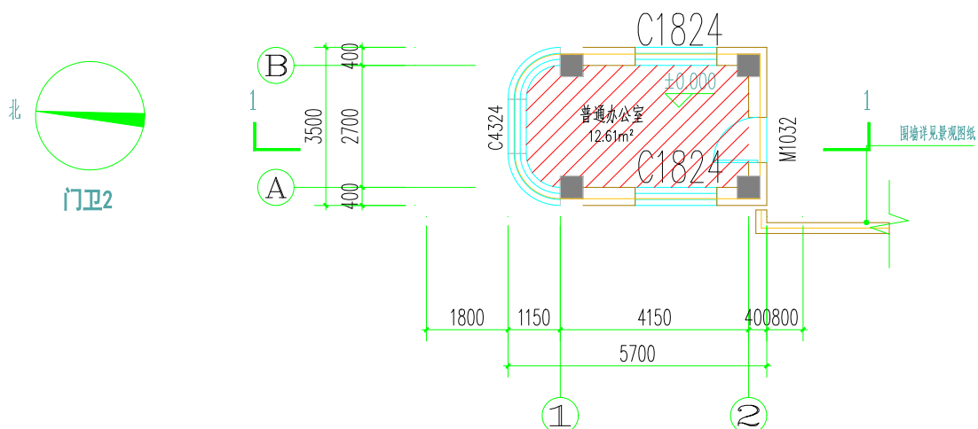
图 5-3 受建筑内设备噪声影响的典型房间楼层平面图
