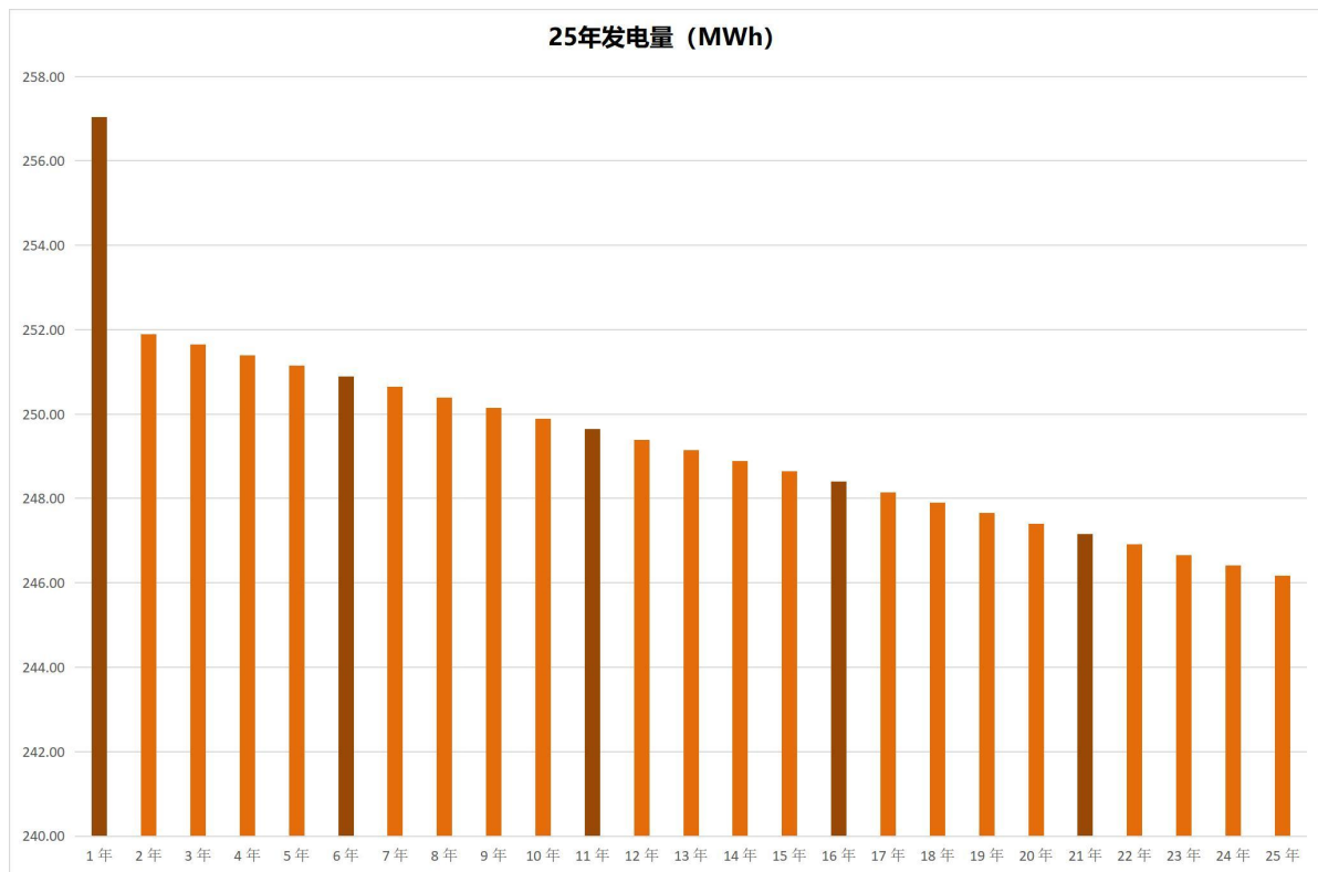
图 12 全周期年发电量
