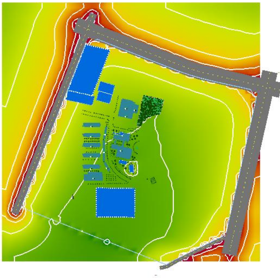
图 5-2 场地 1.5m 高度处声压级分布图（夜间）
