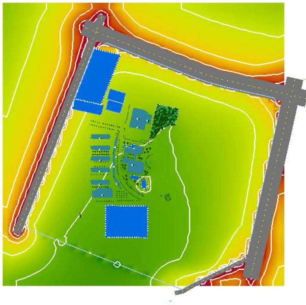
图 4.1-2 场地 1.5m 高度处声压级分布图（夜间）
