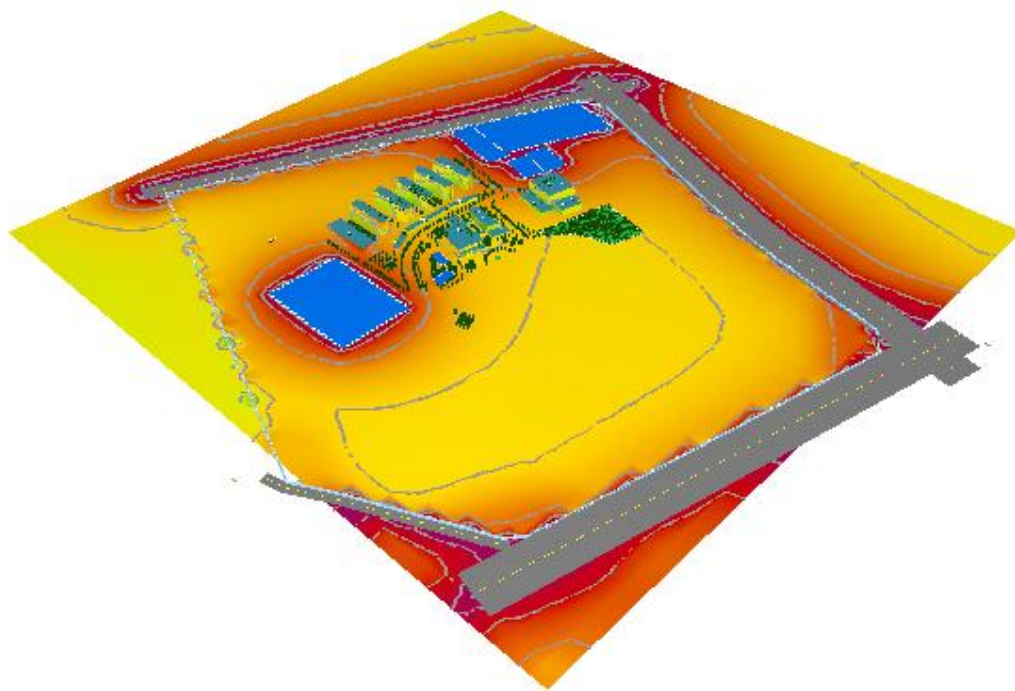
图 4.1-3 场地噪声分布俯瞰图（昼间）
