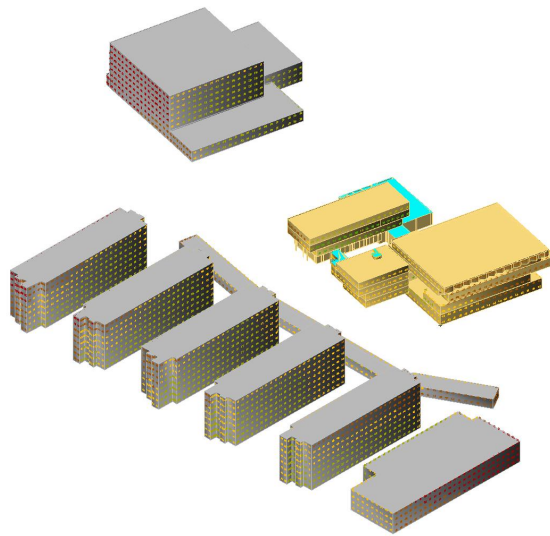
图 4.2-3 参评建筑附近区域声压级鸟瞰分布图（昼间）
