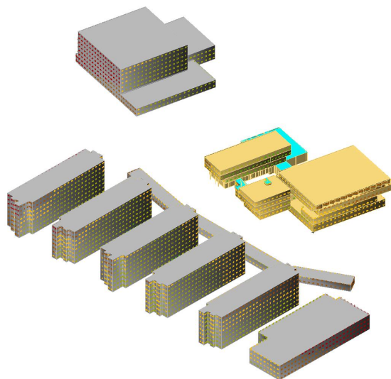
图 4.2-4 参评建筑附近区域声压级鸟瞰分布图（夜间）
