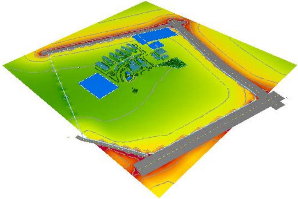
图 4.1-4 场地噪声分布俯瞰图（夜间）
