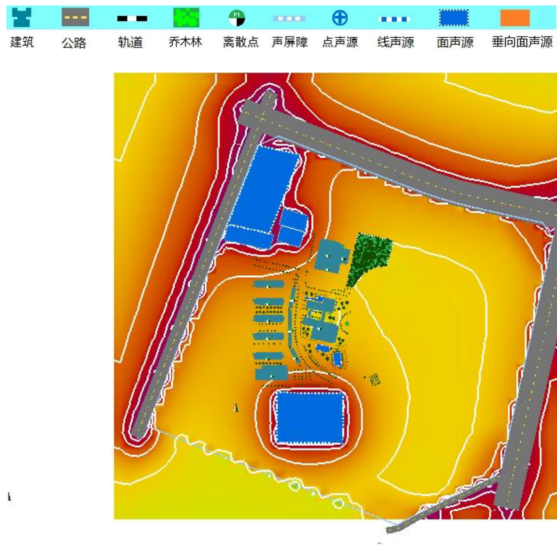
图 4.1-1 场地 1.5m 高度处声压级分布图（昼间）
