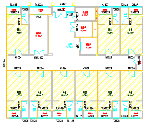
B: 3 层平面
