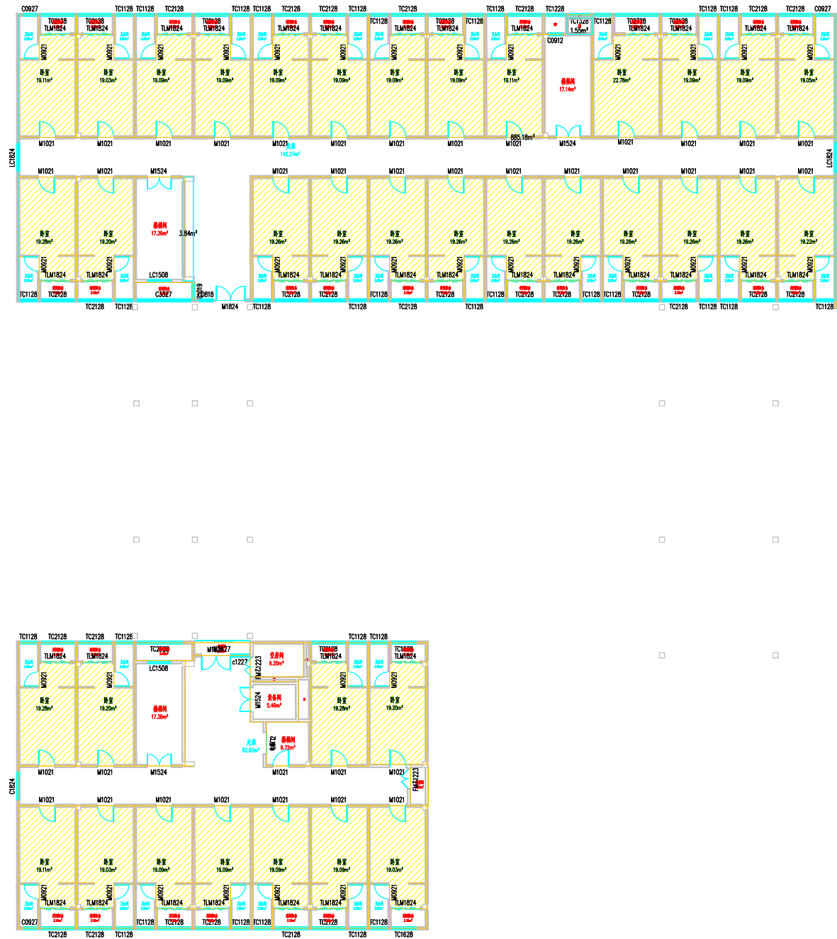
B: 4 层平面
