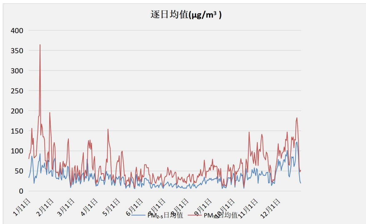
图 5.3 室外颗粒物 PM 2.5 和 PM 10 浓度日均值
