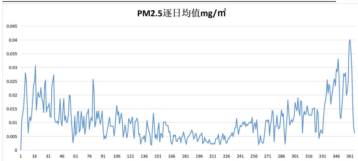
图 6-3 PM 2.5 颗粒物逐日均值图
