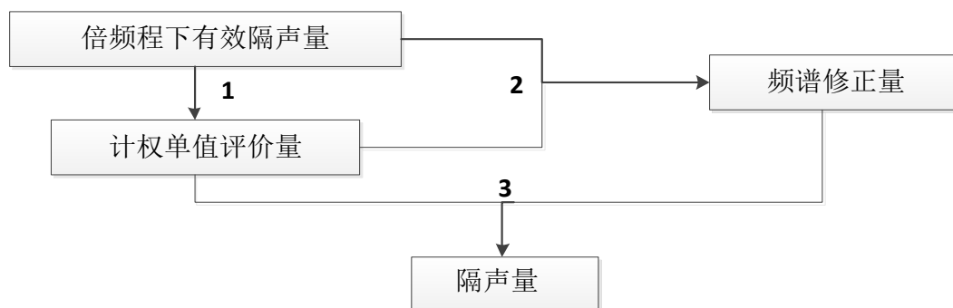
图 7.4-1 组合墙隔声量计算流程图
