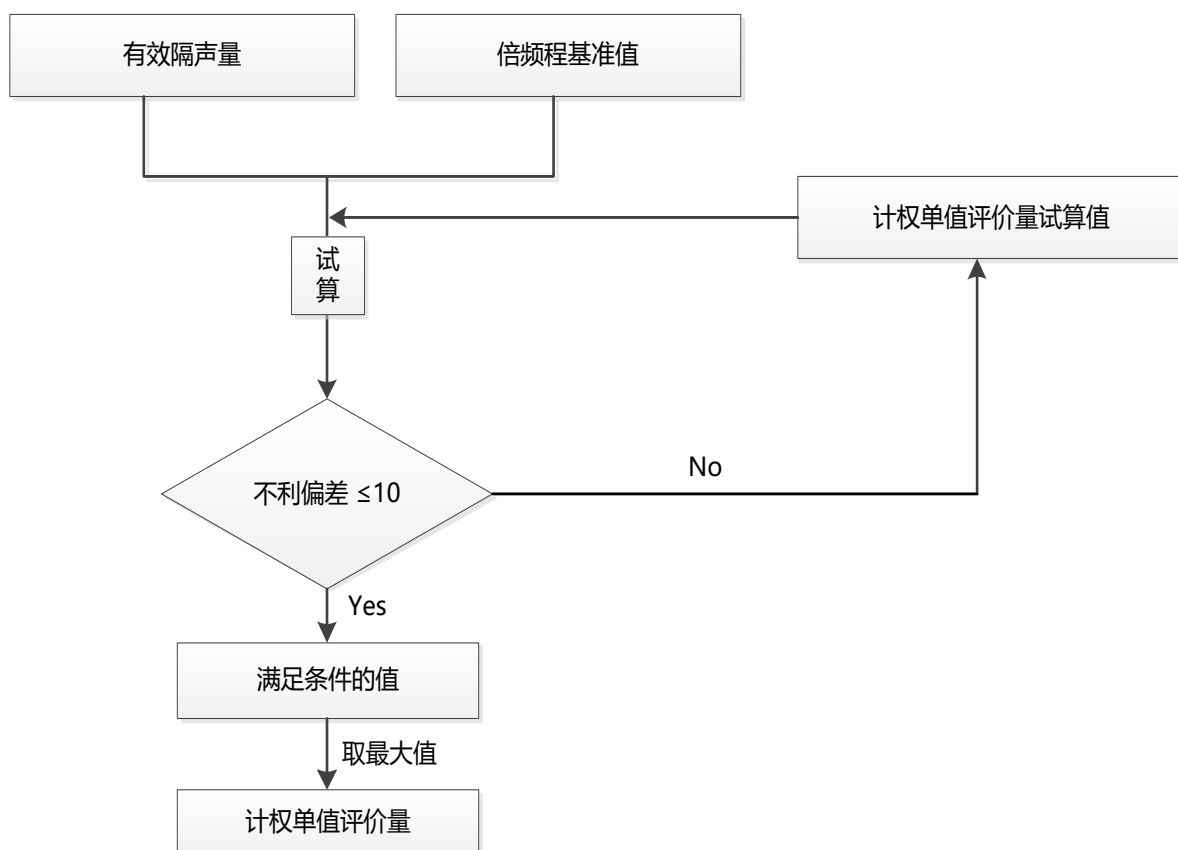
图 7.4.2 组合墙空气声隔声计权单值评价量计算流程
