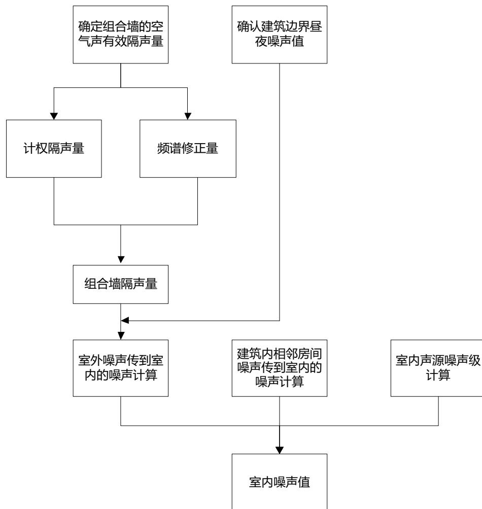
图 5-2 室内噪声级计算原理图
