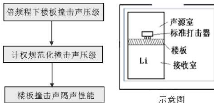
图 7-1 楼板撞击声隔声性能计算过程及测量示意图
