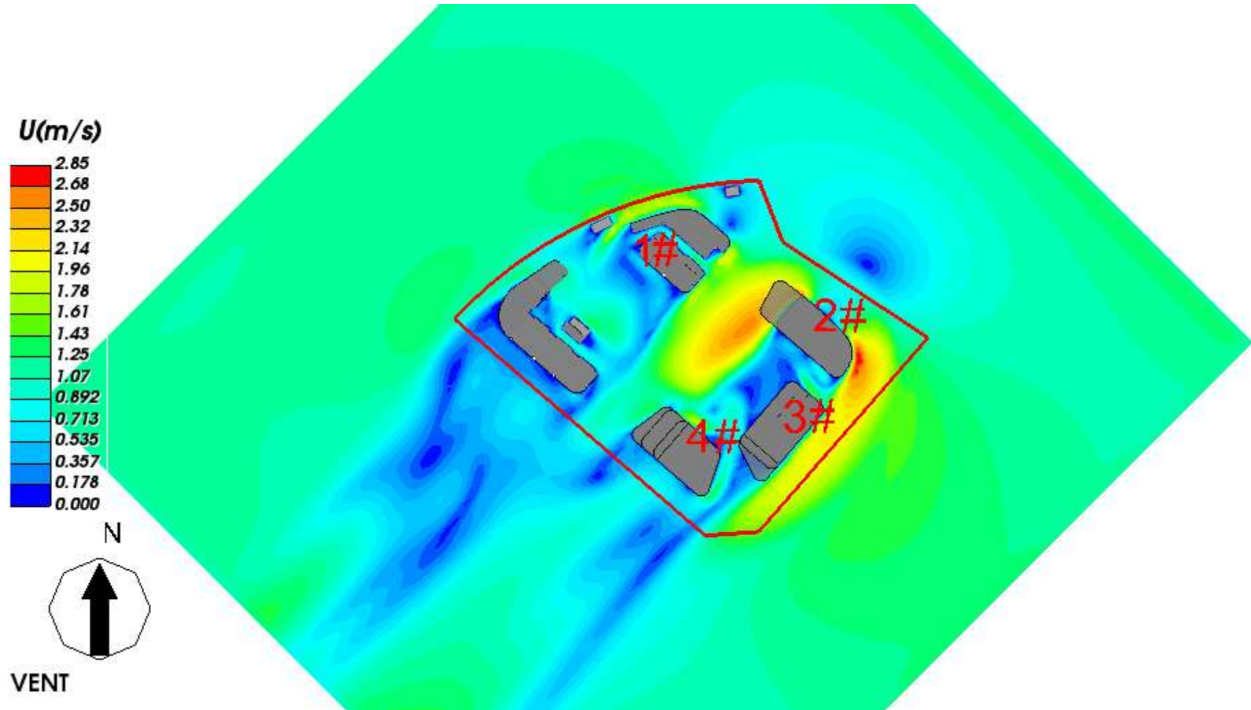
图 5.1-1 1.5 米高处风速云图
