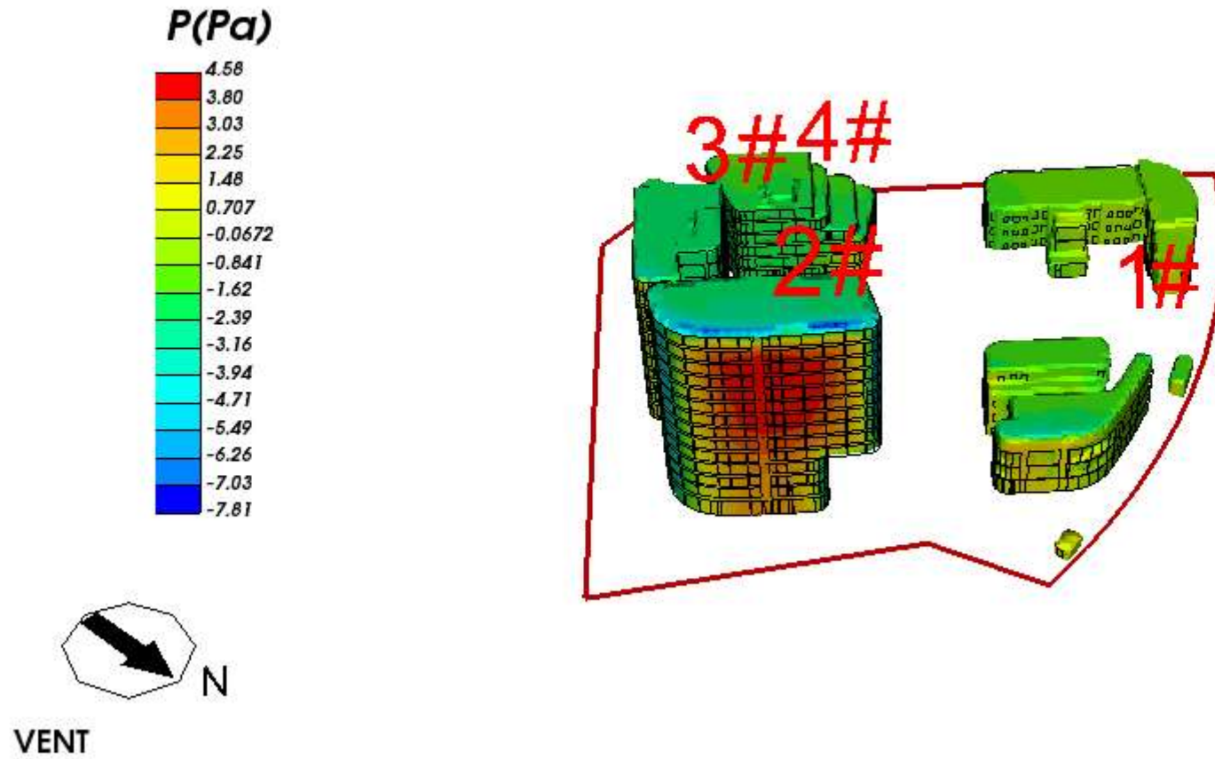
图 5.1-3 建筑迎风面风压云图
