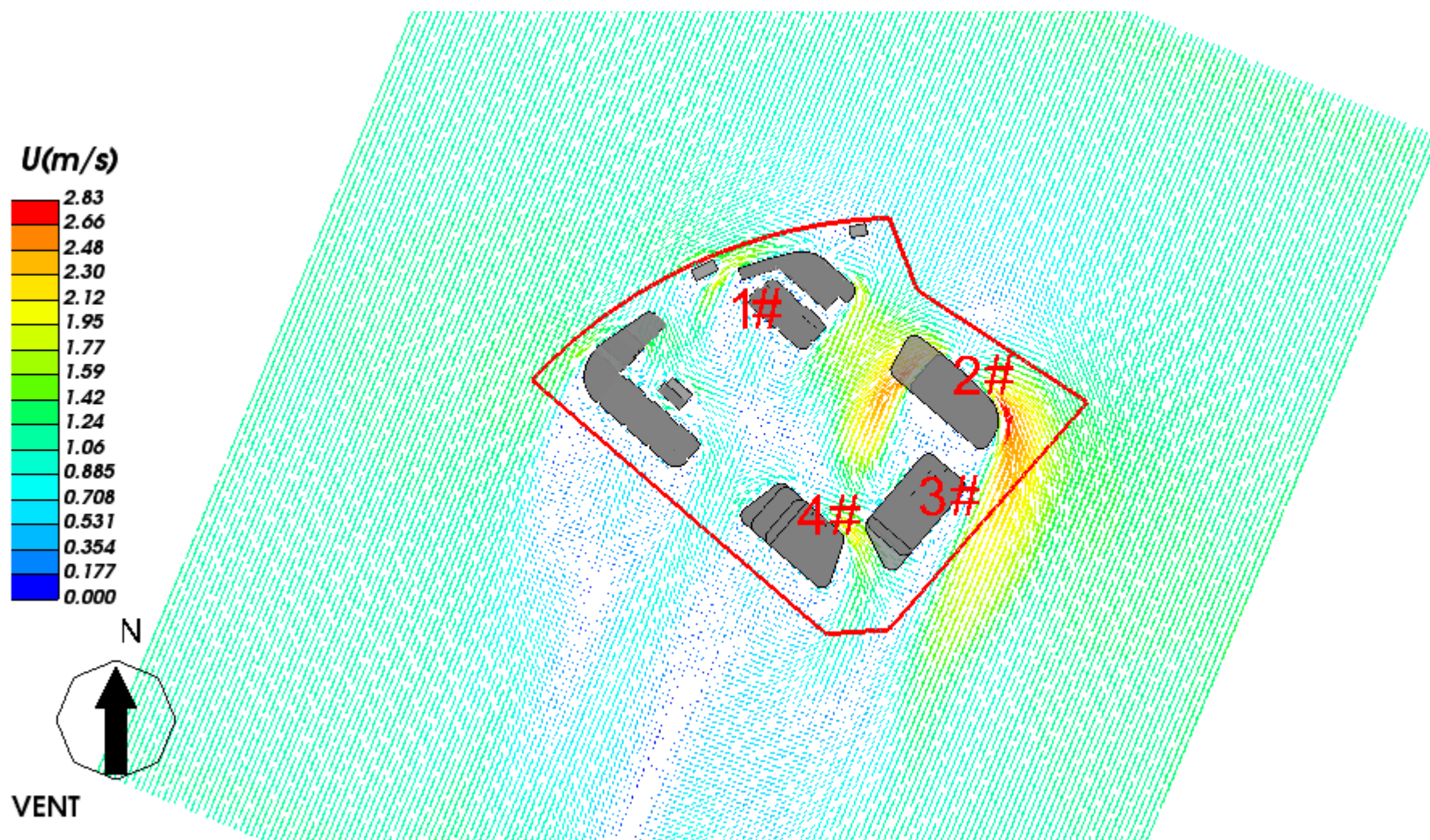
图 5.2-2 1.5 米高处风速矢量图
