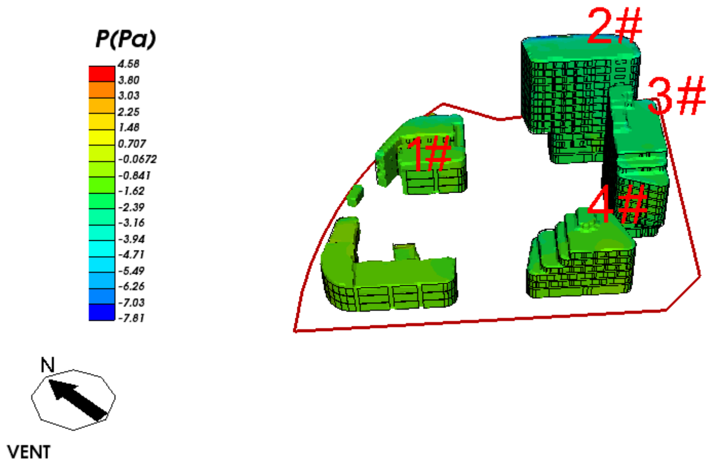
图 5.1-4 建筑背风面风压云图
