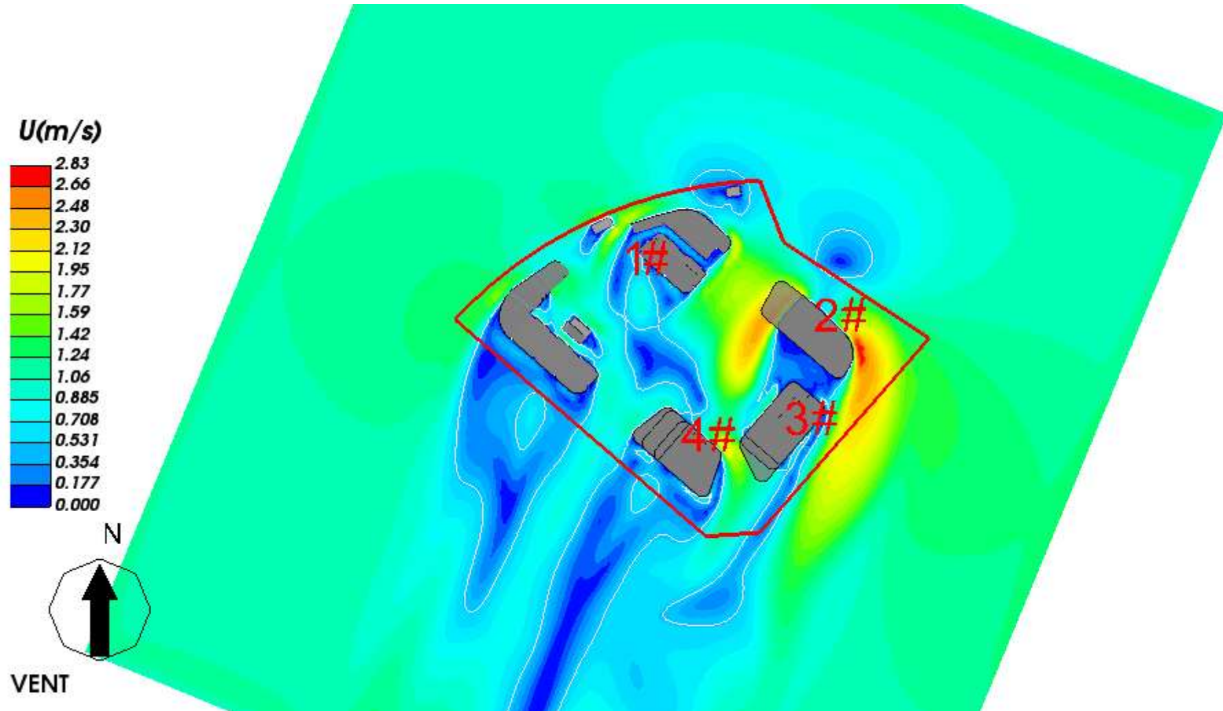
图 5.2-1 1.5 米高处风速云图
