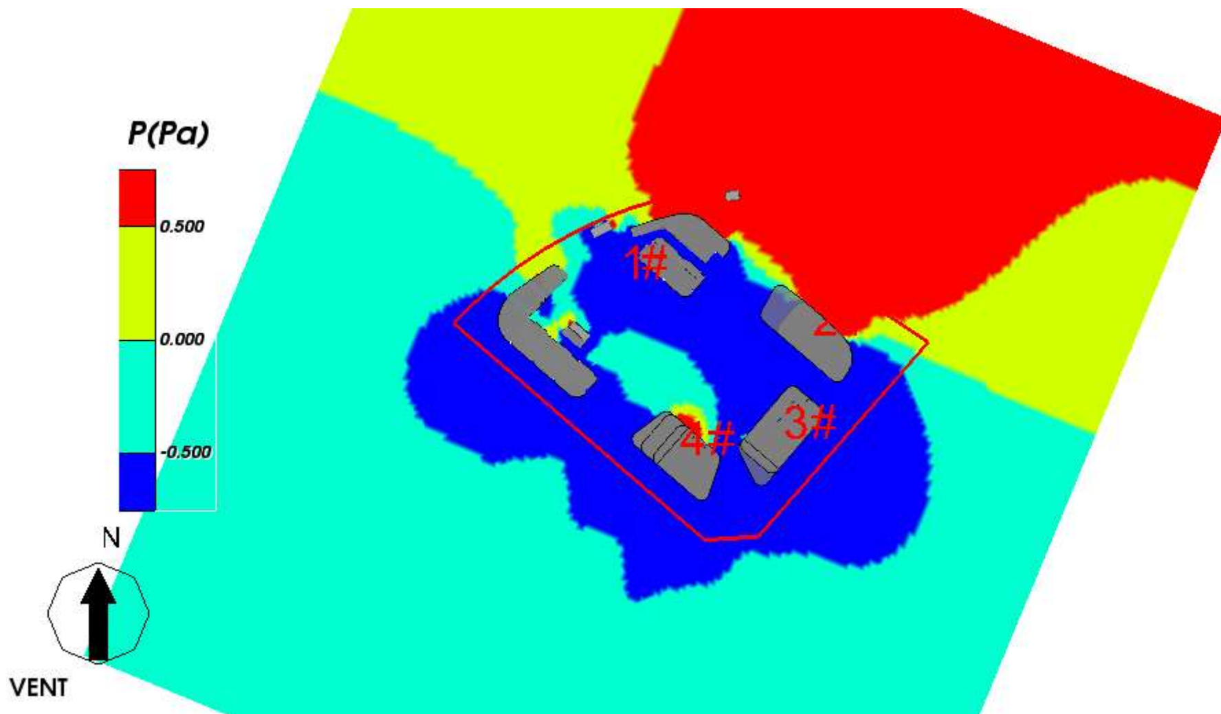
图 5.2-3 1.5 米高处风压云图
