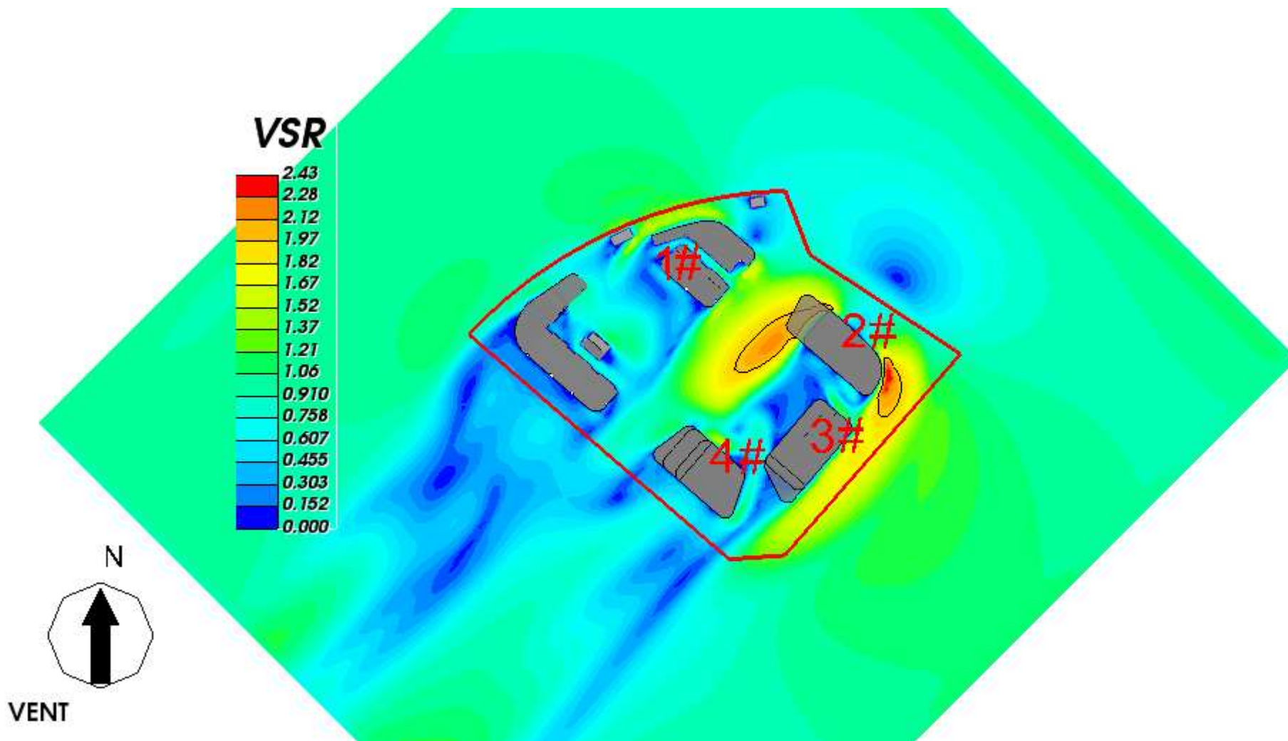
图 5.1-2 1.5 米高处风速放大系数云图
