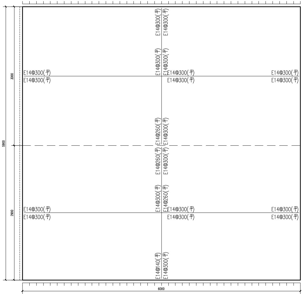
选筋结果(控制工况)
