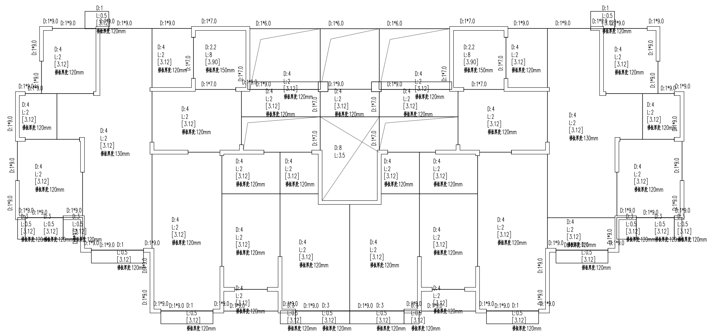
第 17 页 第 5 层平面图 [ 单位: m ] [ D: 面积 L: 面积 R: 面积 ]
