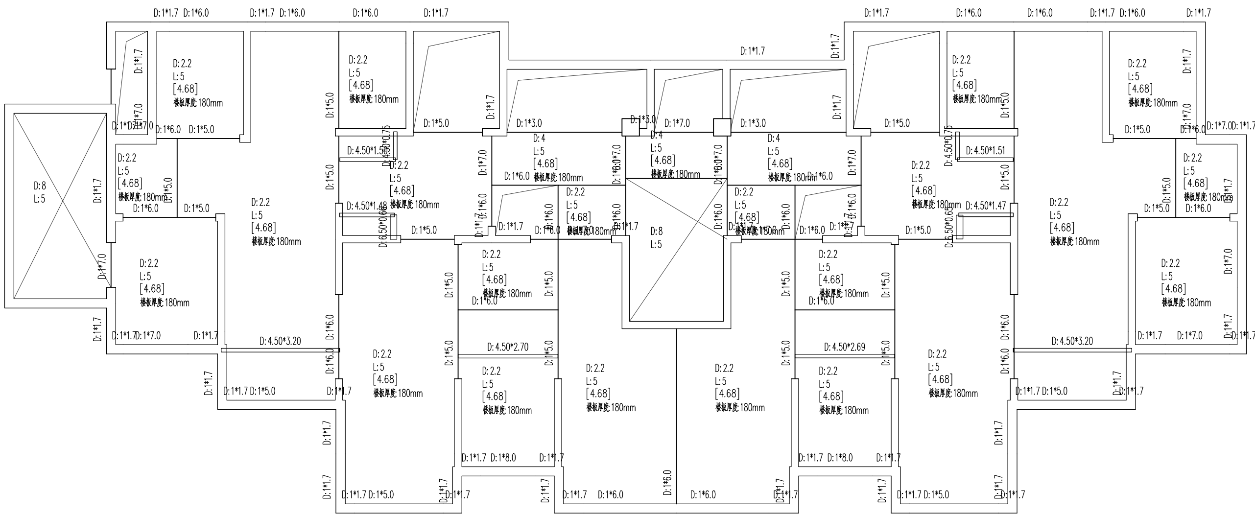
第2 层(第2 标准层)的图。注：节点编号为楼层号 [ 单位:MM, m ] [ D:轴号 L:轴号 R:人防轴号 ] 注:人防轴号
