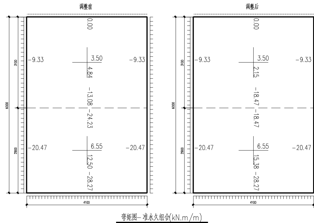
准永久组合弯矩图
