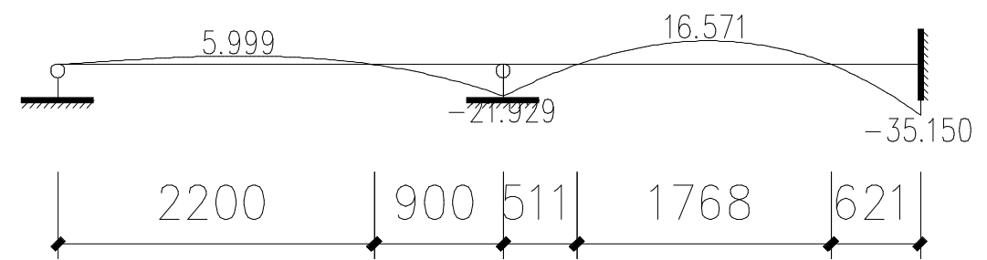
竖向弯矩图-准永久组合(kN.m/m)
