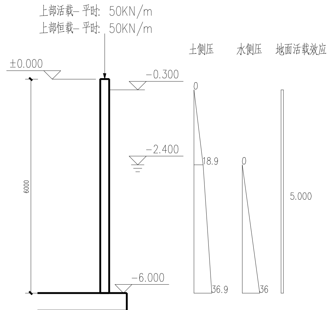
荷载图
