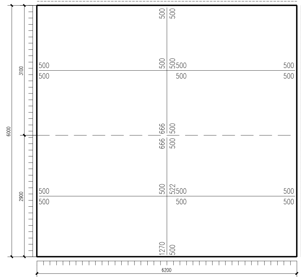
计算配筋面积简图-平时组合(mm 2 /m)
