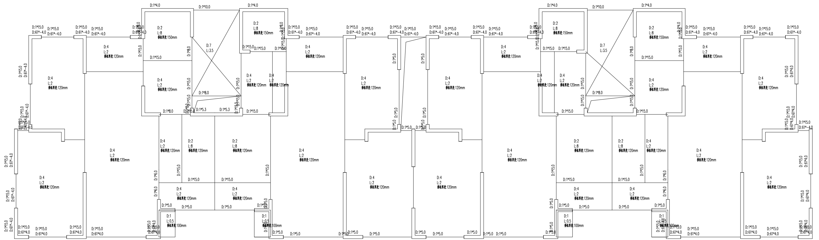
第 20 层(第 6 标准层)楼、墙、柱、剪力墙截面荷载 [ 单位:kN.m ] [ D:恒载 L:活载 R:人防荷载 [ ] 中为楼面自重 ]
