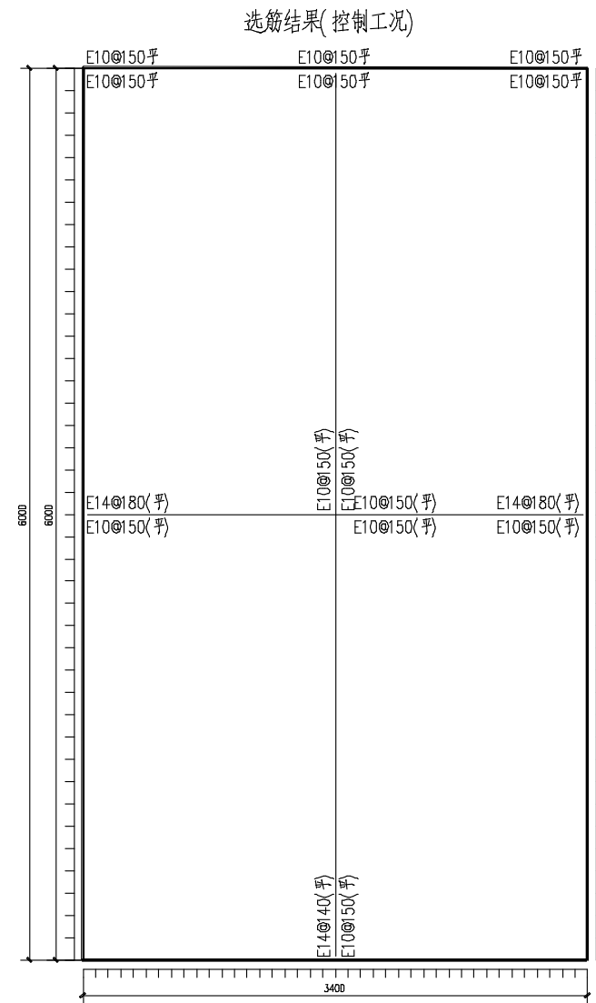
实际配筋简图
