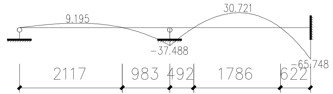
竖向弯矩图-平时组合(kN.m/m)
