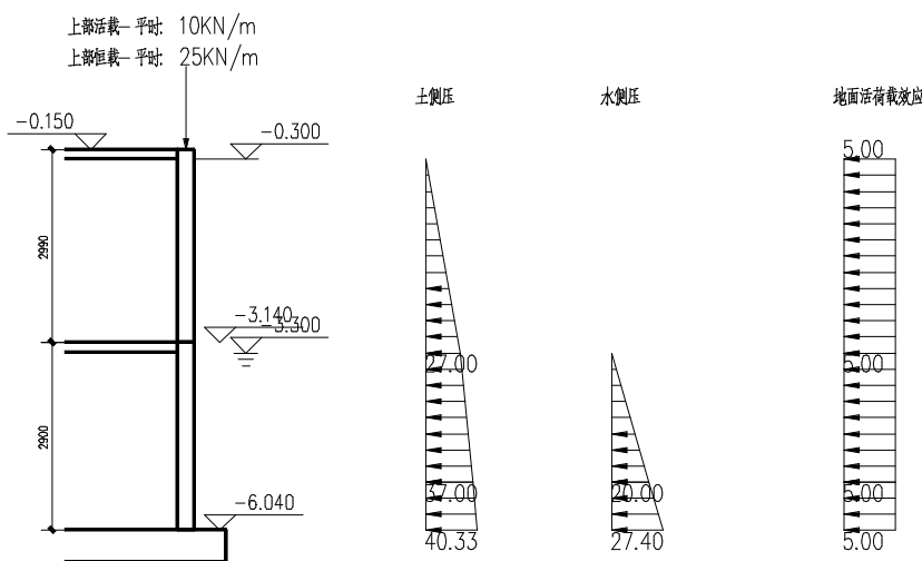
荷载图
