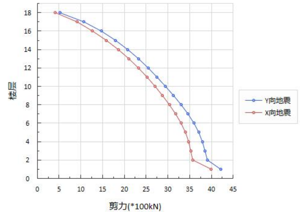
图 6-9 地震作用下楼层剪力简图(塔 1)
