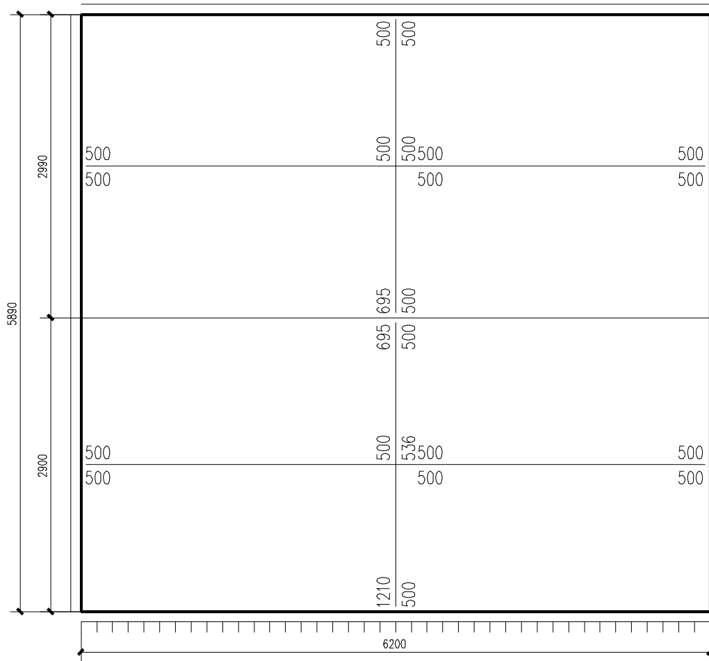
计算配筋面积简图—平时组合(mm 2 /m)
