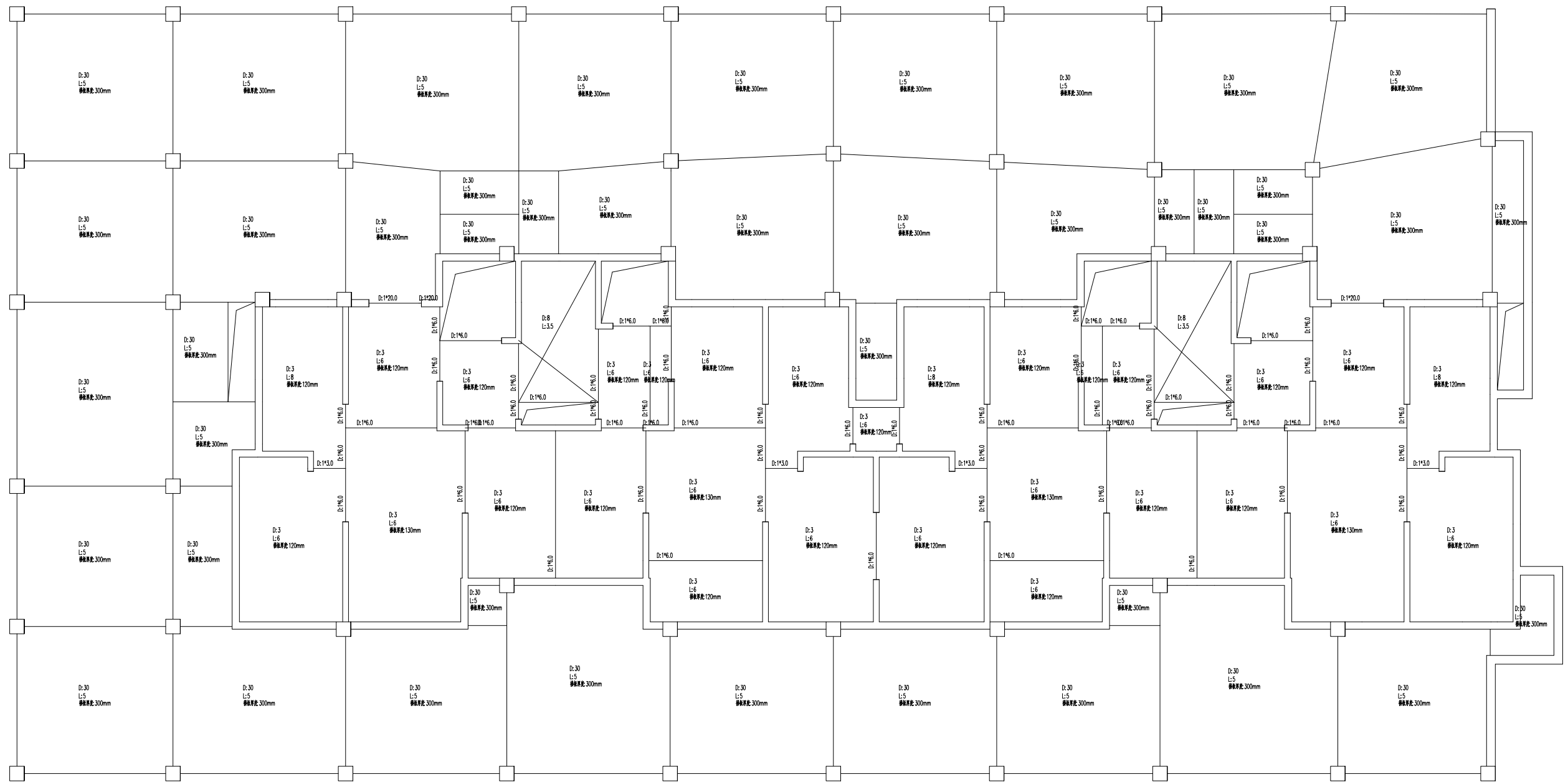
第 1 层(第 1 层)荷载简图 [单位: kN/m] [D:恒载 L:活载 R:人防荷载 [人防荷载按图]]
