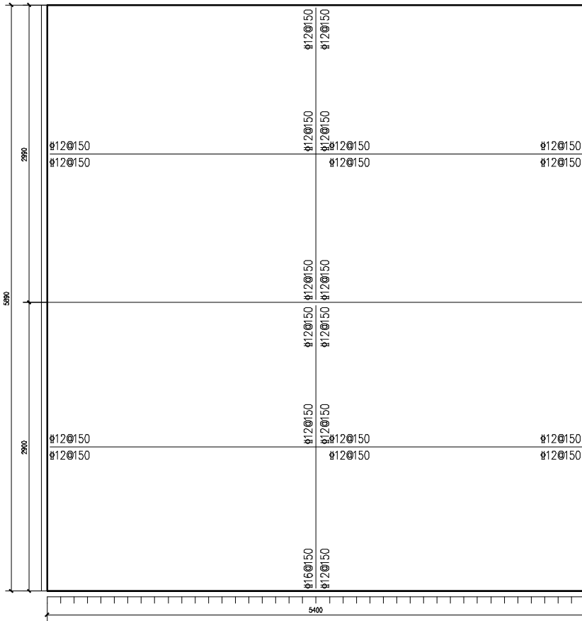
实际配筋简图
