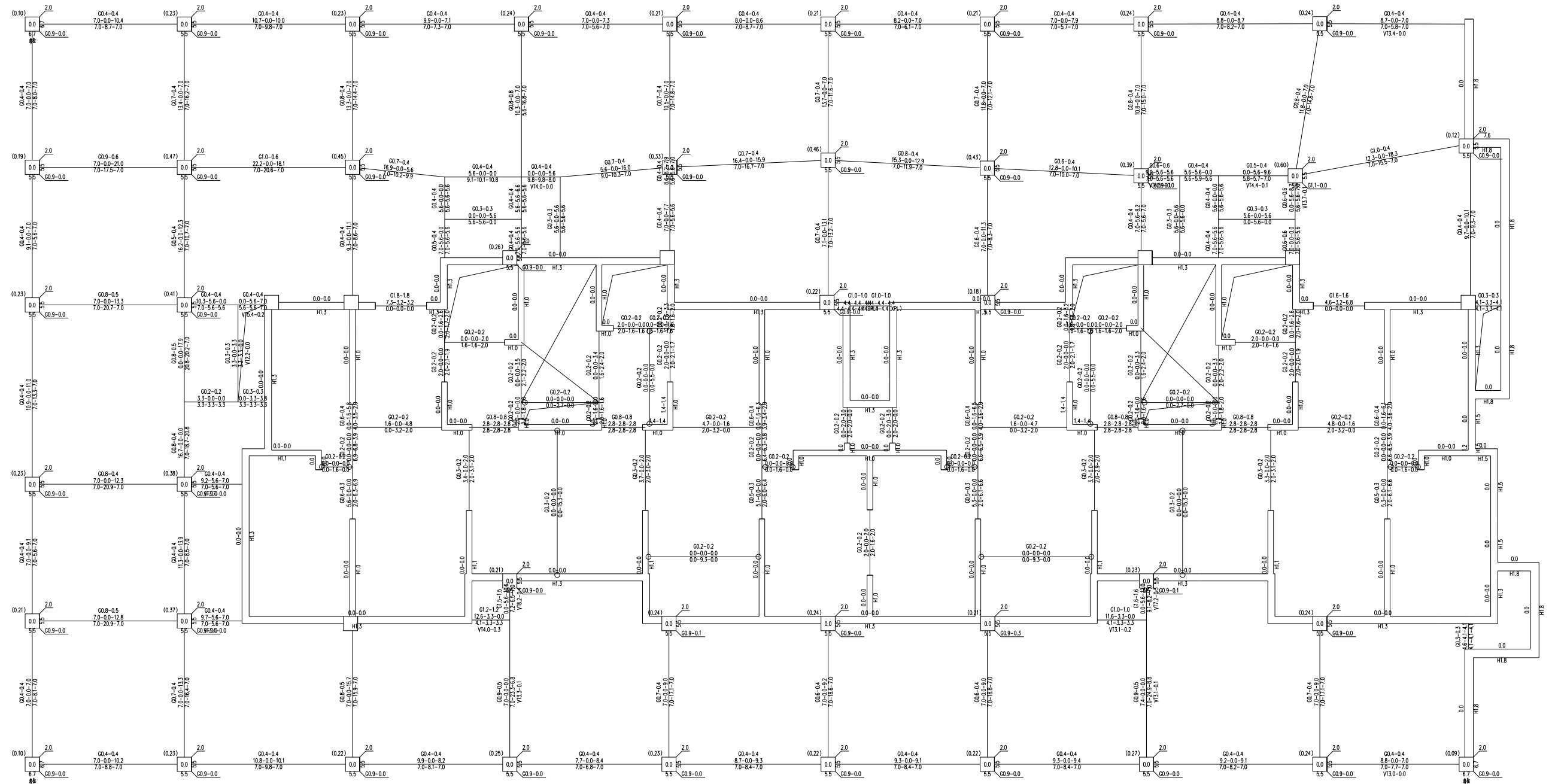
第 1 层(标准层1 地下2层) 混凝土构件配筋及钢筋应力比简图(单位:cm 2 ) 层高=2900(mm) 梁总数=156 柱总数=50 墙柱总数=83 混凝土强度等级 梁Cb=C30 柱Cc=C30 墙Cw=C30 主筋强度 梁Fb=360 柱Fc=360 墙Fw=360 箍筋(分布筋)强度 梁=360 柱=360 墙水平=360 墙竖向=360 过墙柱=360 箍筋间距(mm): 梁=100 柱=100 墙水平分布筋间距=200(mm),墙竖向分布筋配筋率=0.25%
