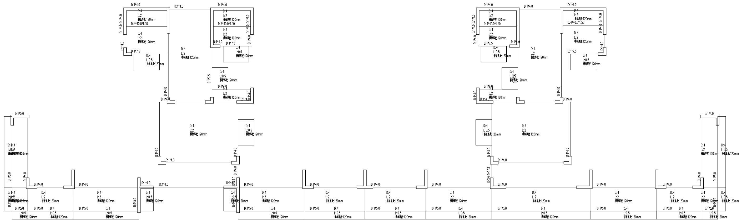
第 18 层(第 7 标准层)梁、柱、字高荷载平面简图 [ 单位:kN·m ] [ D:板载 L:活载 R:人防荷载 [ ]中为转换层梁 ]
