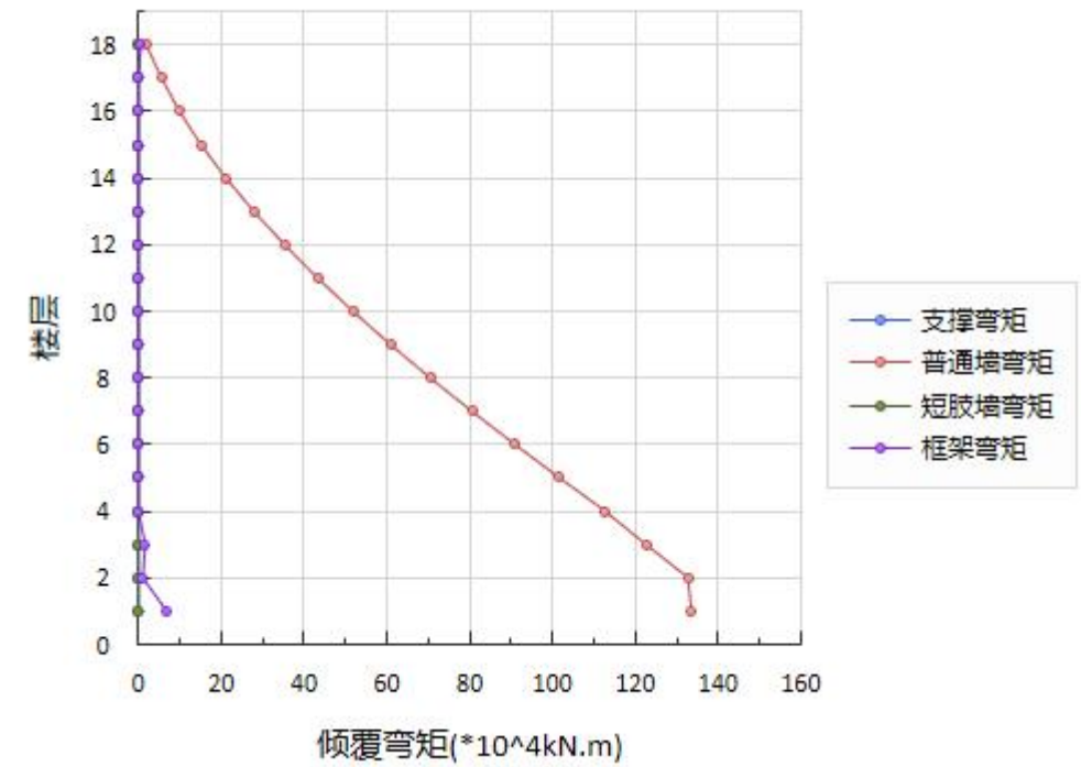
图 6-4 Y 静震下倾覆力矩简图(塔 1)
