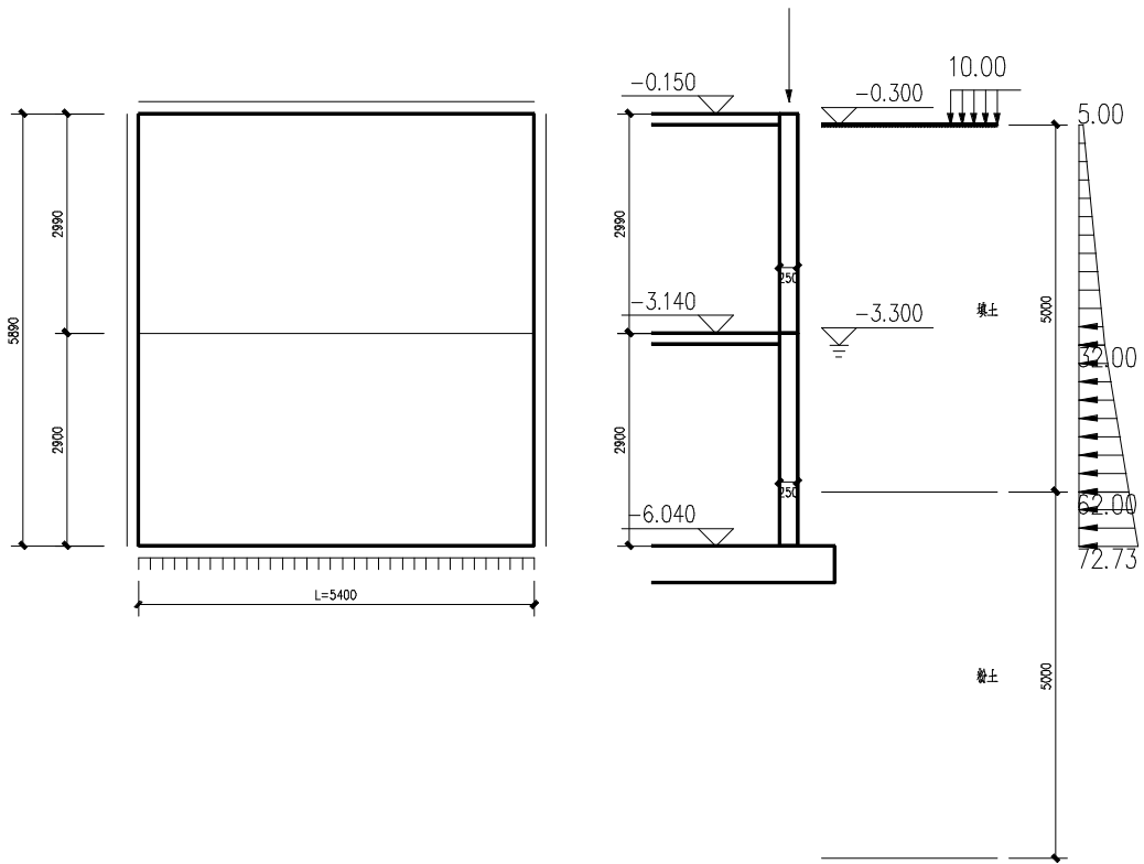
外墙尺寸模型简图
