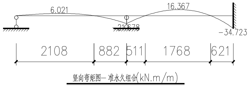
准永久组合弯矩图
