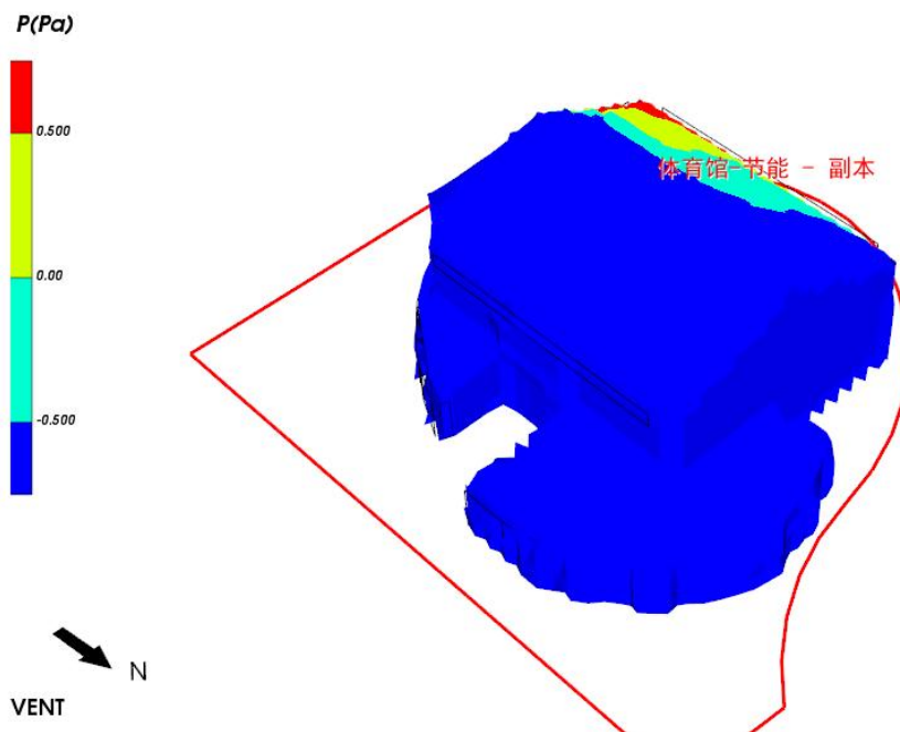
图 5.4- 2 建筑背风面外窗表面风压云图-过渡季
