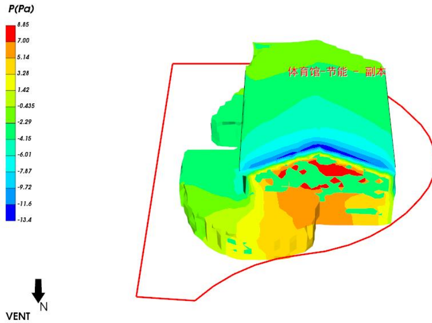
图 5.2- 4 建筑迎风面风压云图
