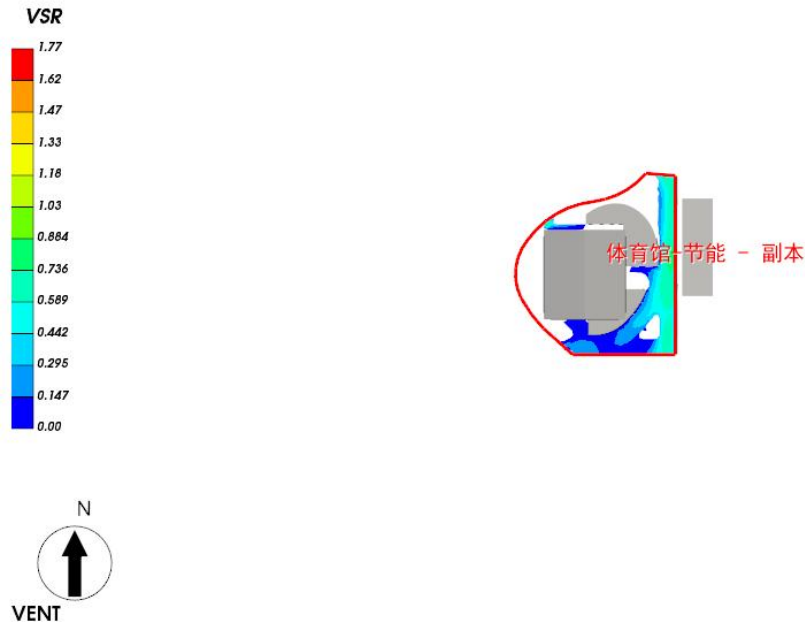
图 5.2- 2 人行区域-1.5 米高度水平面风速放大系数云图-冬季
