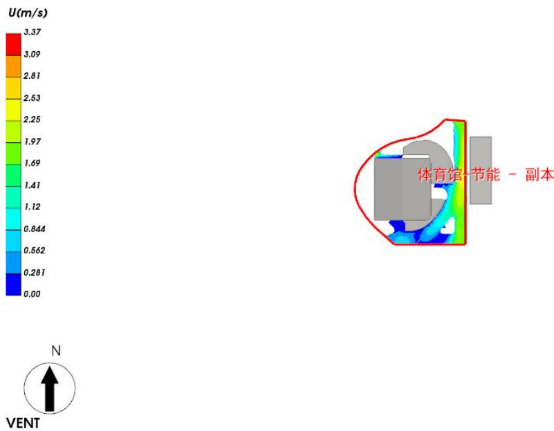
图 5.2- 1 人行区域-1.5 米高度水平面风速云图-冬季
