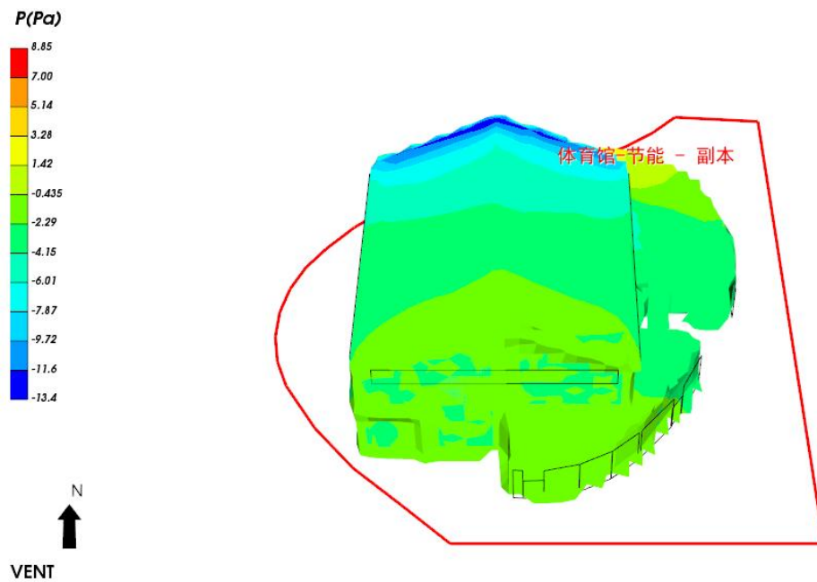
图 5.2- 5 建筑背风面风压云图
