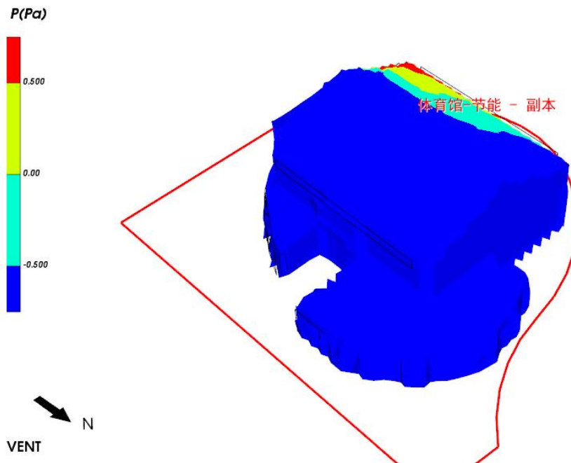
图 5.3- 2 建筑背风面外窗表面风压云图-夏季
