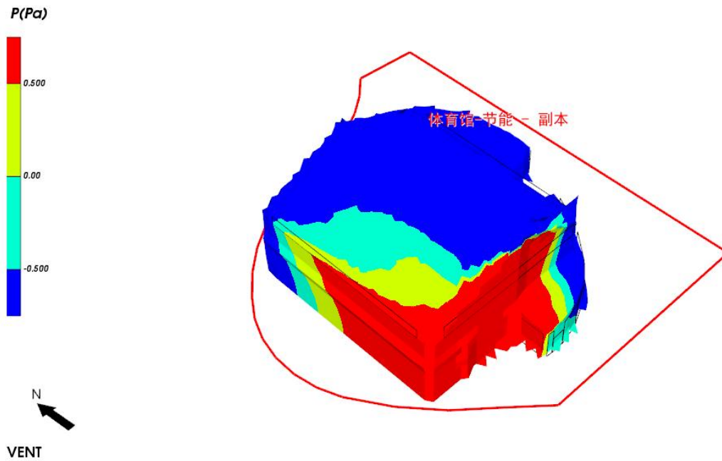
图 5.4- 1 建筑迎风面外窗表面风压云图-过渡季
