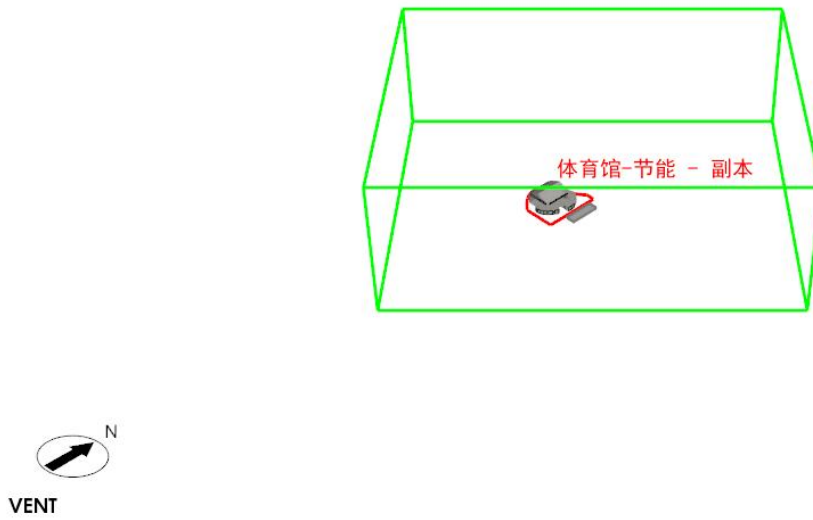
图 4.11 夏季工况风场计算域图示
