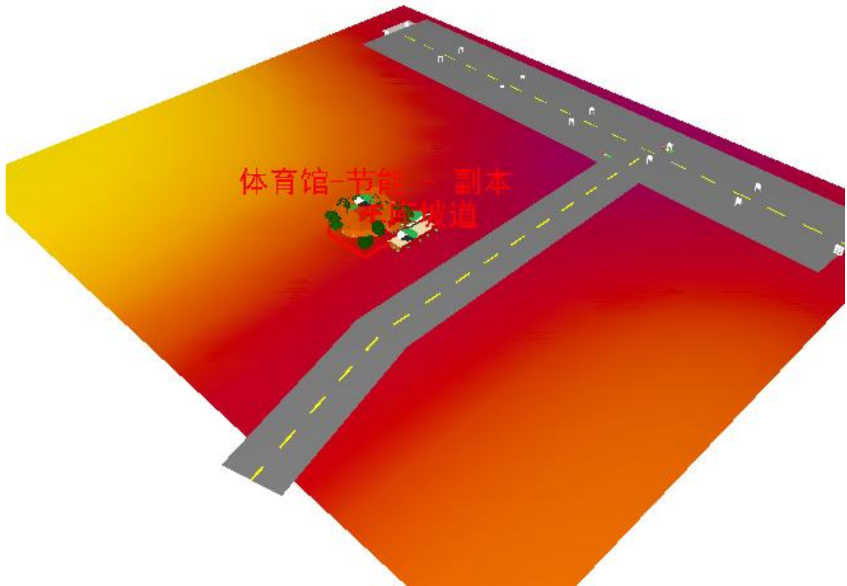
图 4.1-3 场地噪声分布俯瞰图（昼间）
