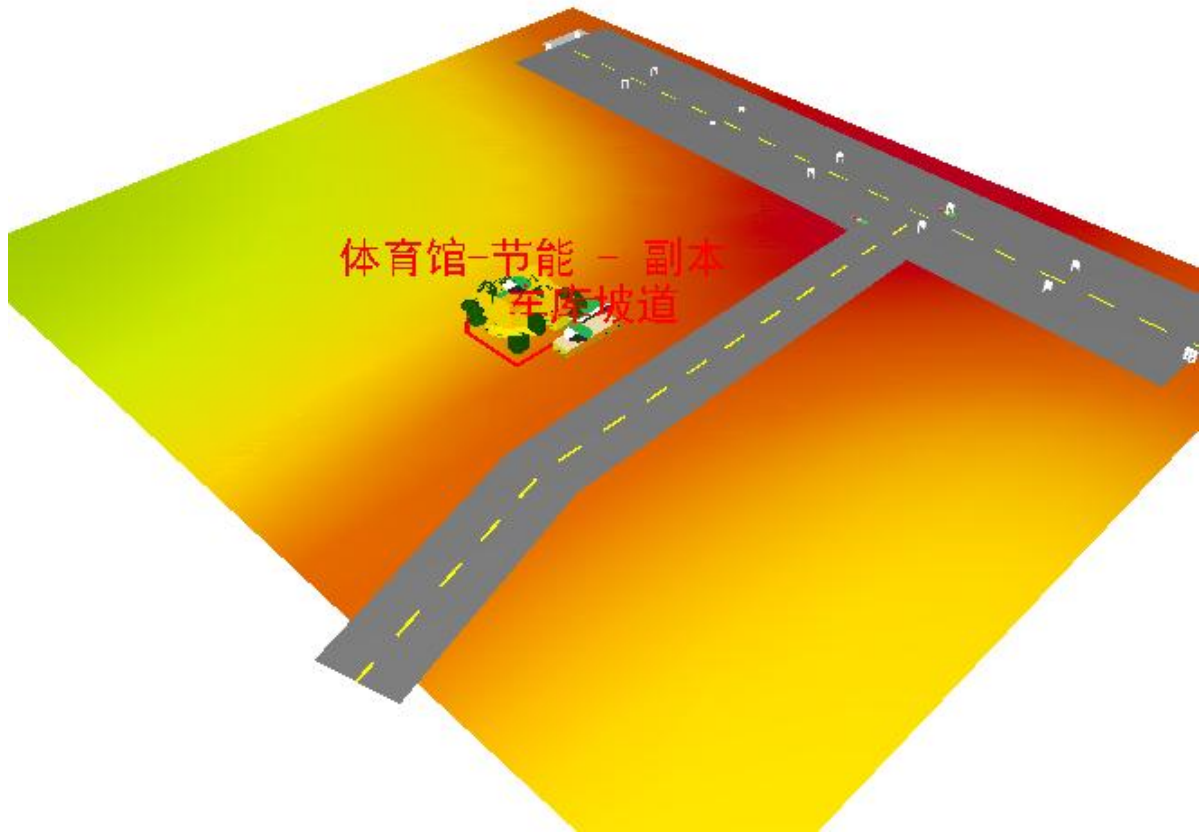
图 4.1-4 场地噪声分布俯瞰图（夜间）
