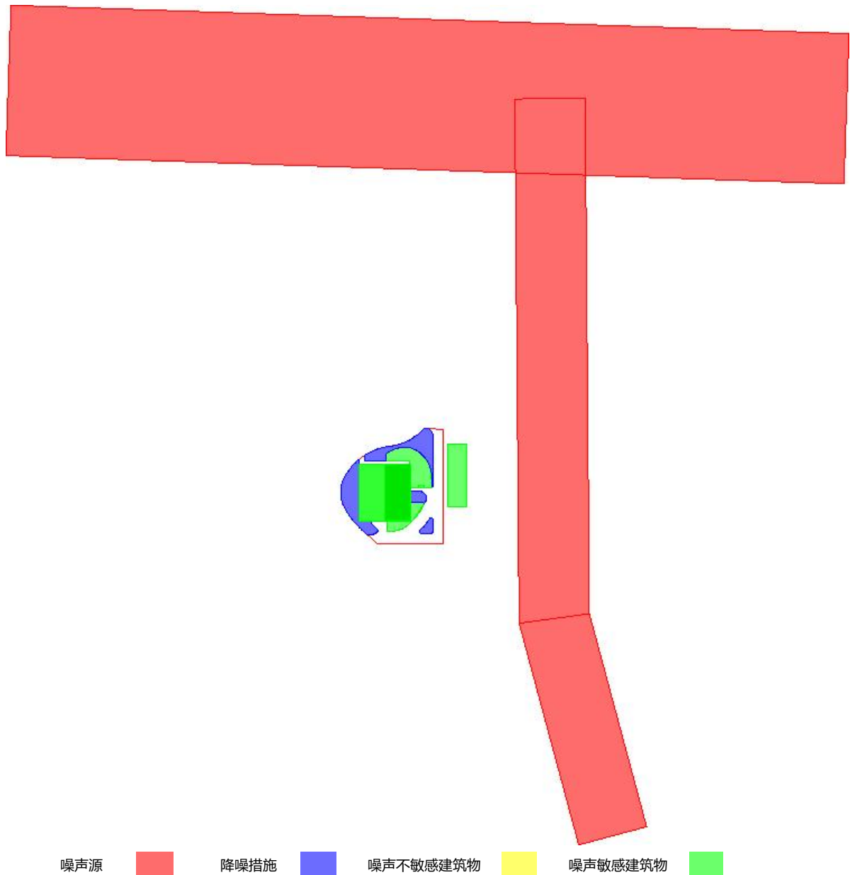
图 3.2-2 室外声区标注图
