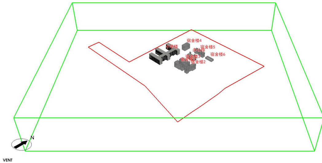
图 4.11 冬季工况风场计算域图示
