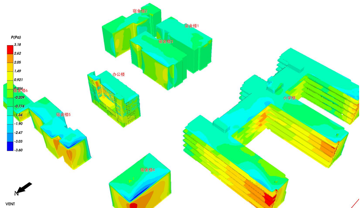
图 5.2- 4 建筑迎风面风压云图
