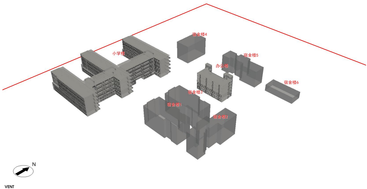
图 4.11 夏季工况风场计算域图示
