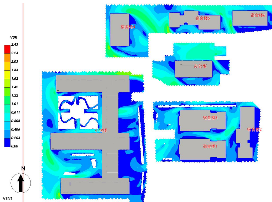
图 5.2- 2 人行区域-1.5 米高度水平面风速放大系数云图-冬季
