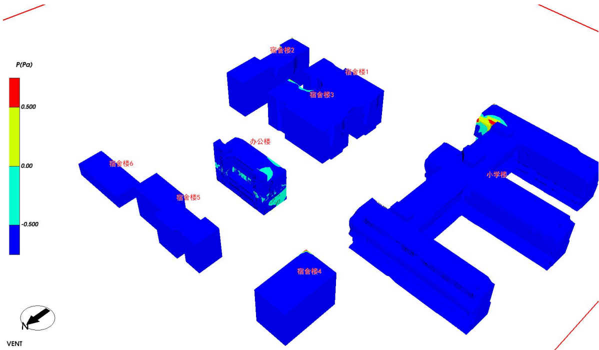
图 5.3- 2 建筑背风面外窗表面风压云图-夏季
