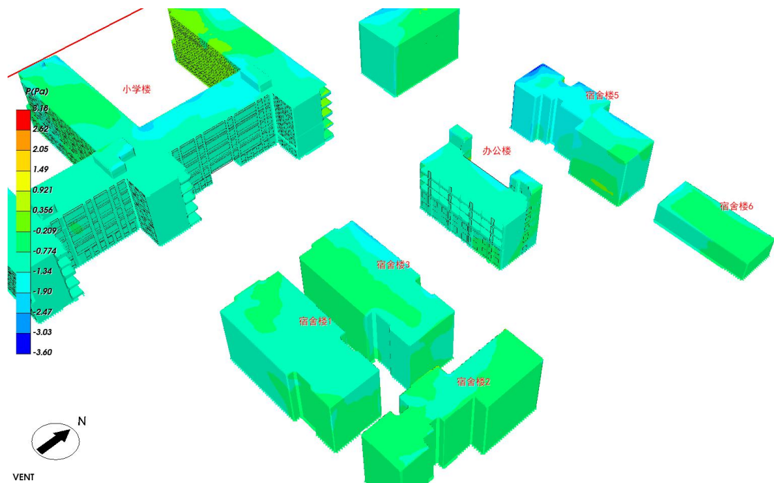
图 5.2- 5 建筑背风面风压云图
