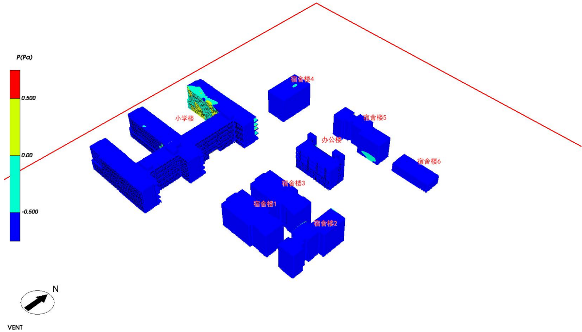
图 5.4- 2 建筑背风面外窗表面风压云图-过渡季
