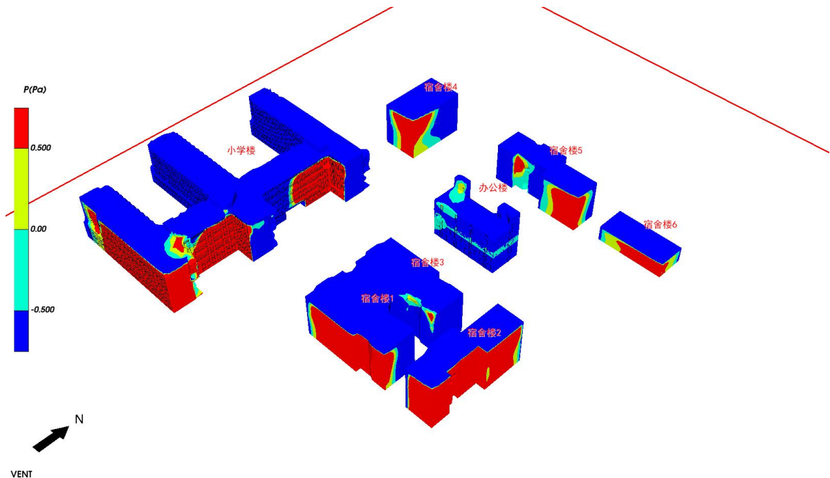
图 5.3- 1 建筑迎风面外窗表面风压云图-夏季
