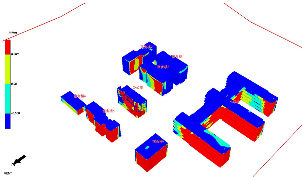
图 5.4- 1 建筑迎风面外窗表面风压云图-过渡季
