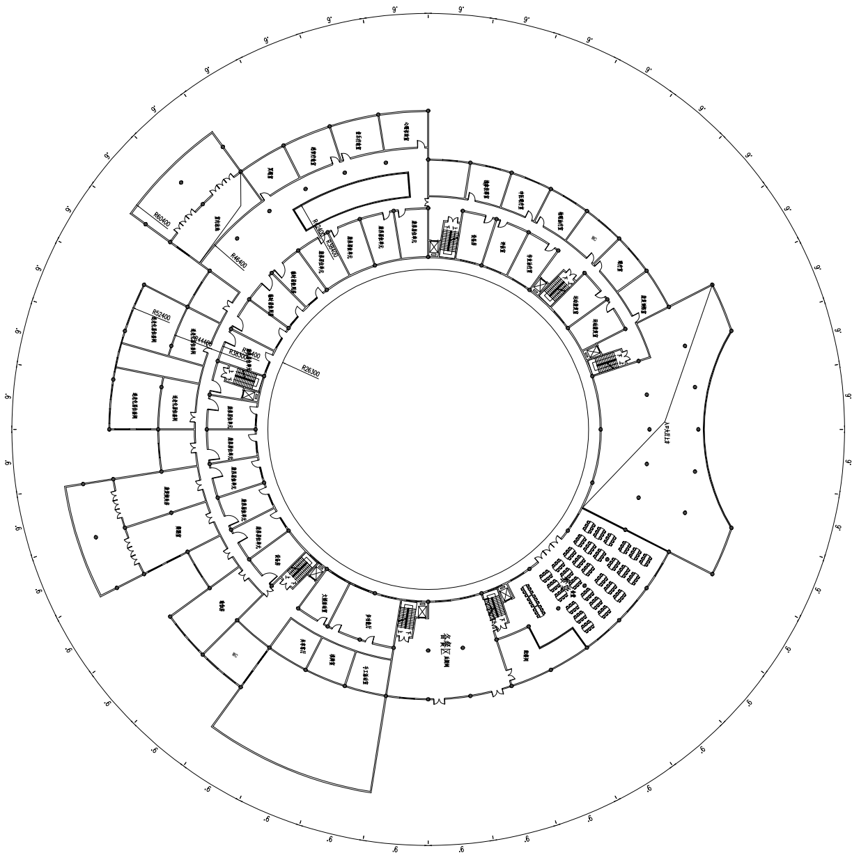
一层平面图: 200
