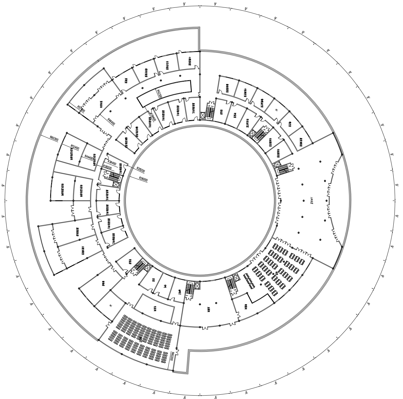
首层平面图 1:200
