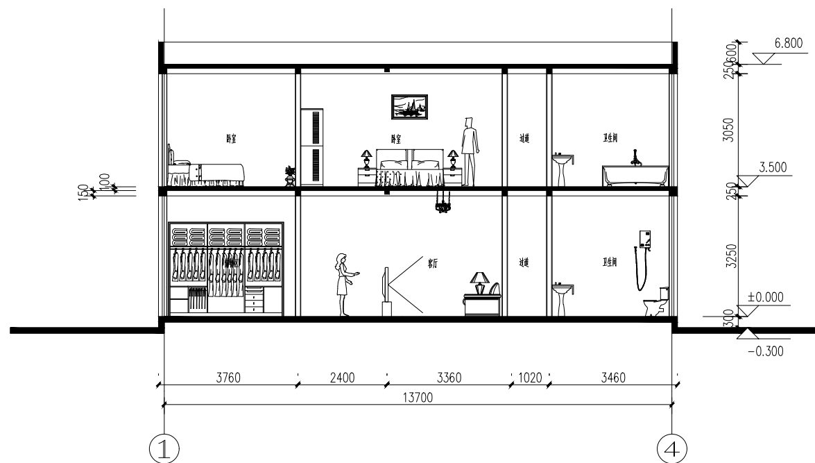
剖面图1-1 1:100
