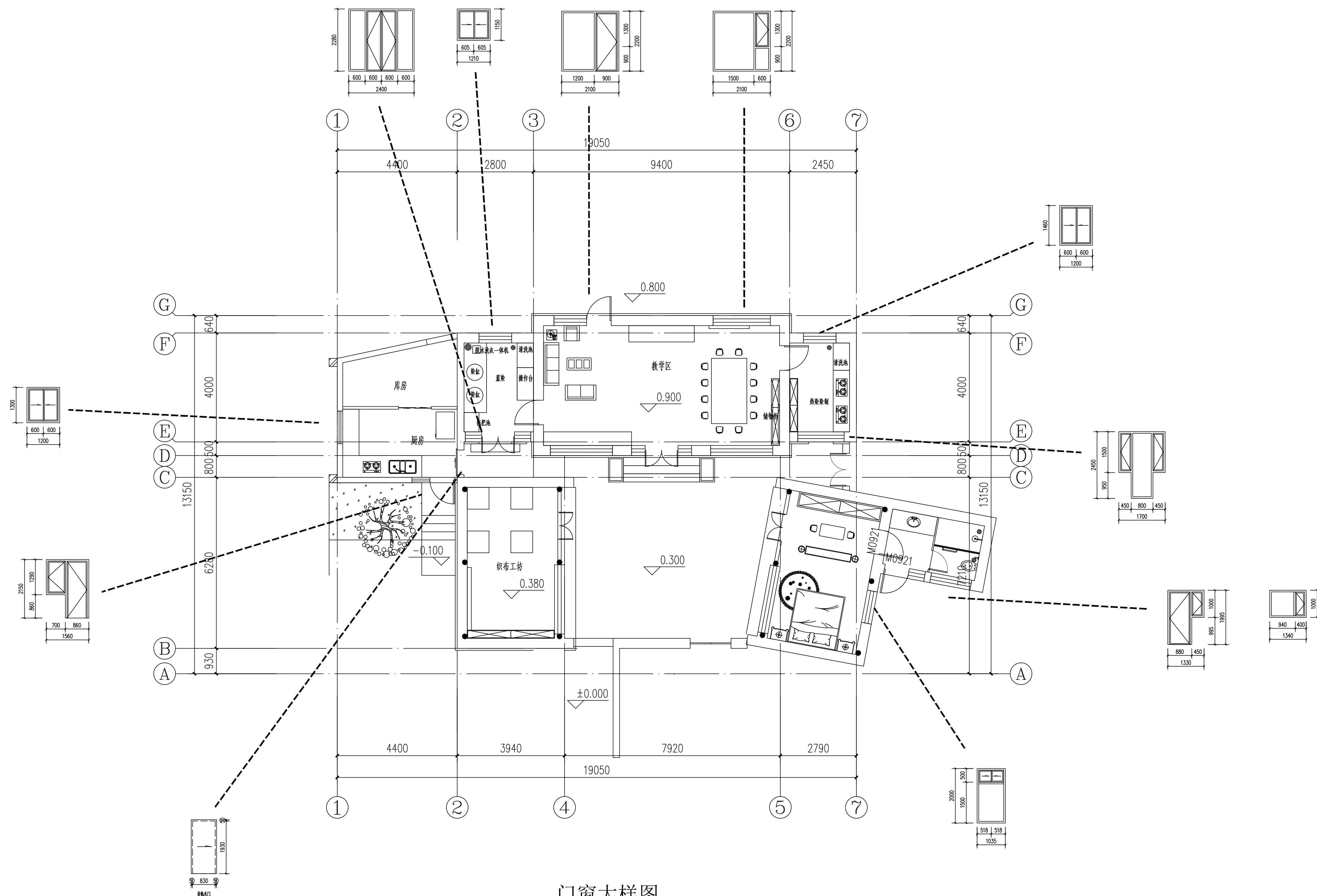
门窗大样图
