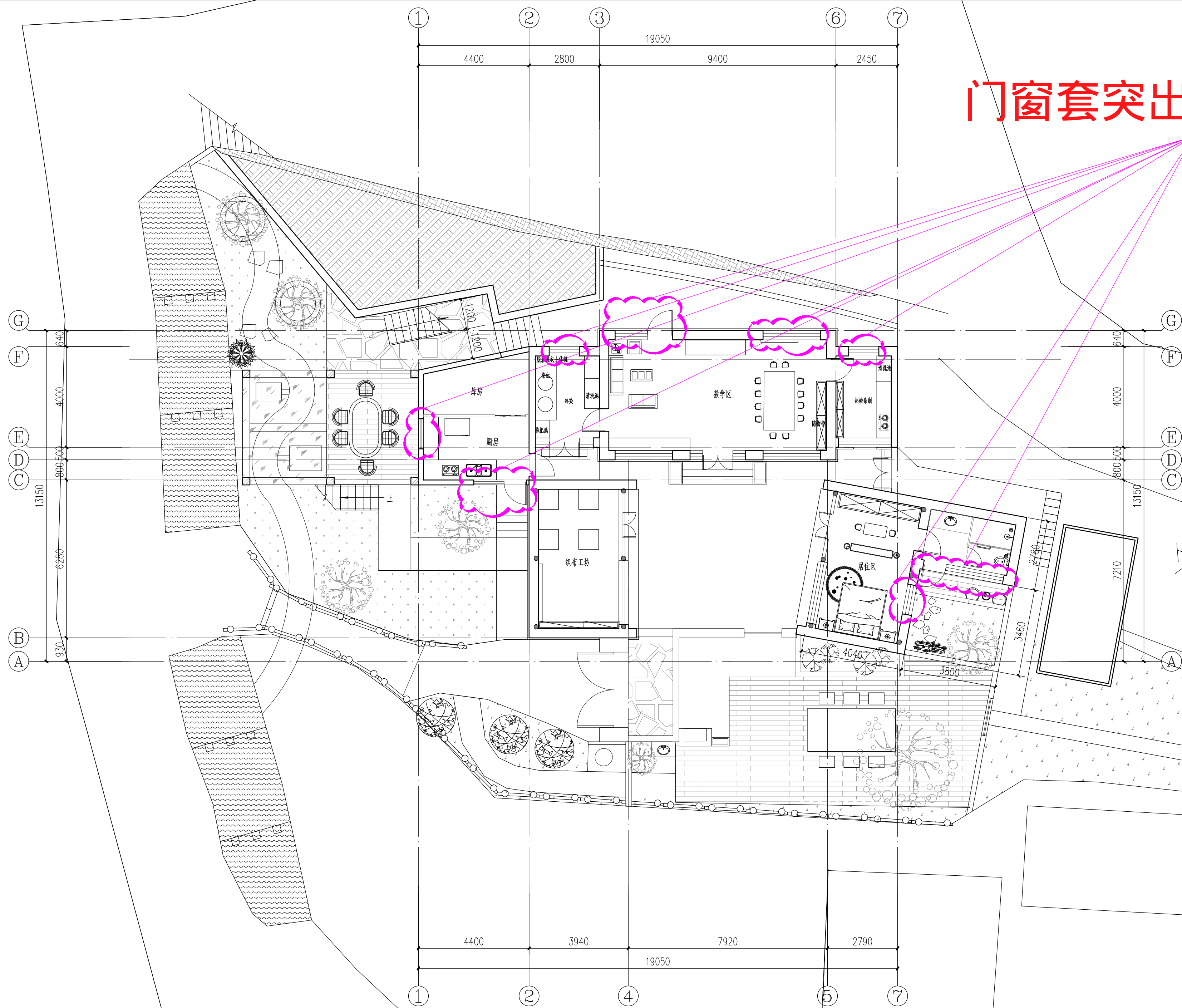
一层平面图 1:100
