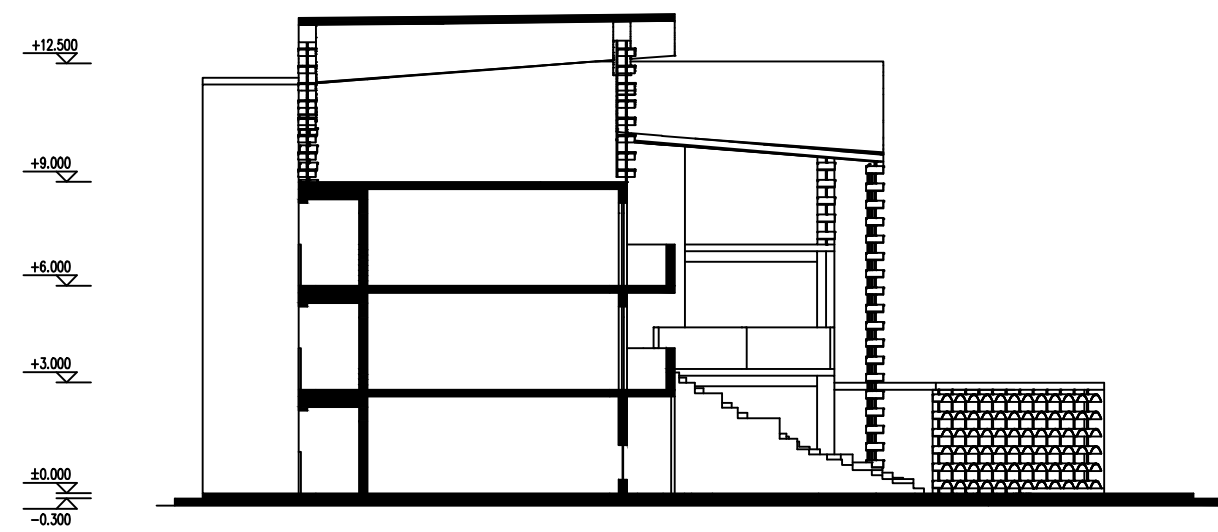
剖面图 1: 200
