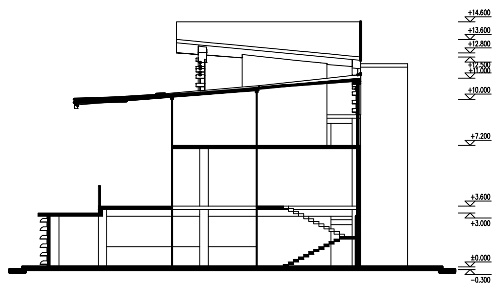
剖面图 1: 200
