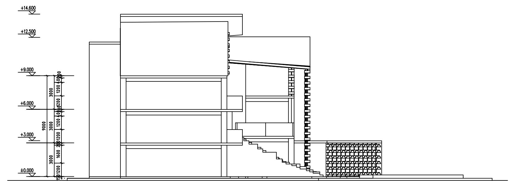
西立面图 1: 200
