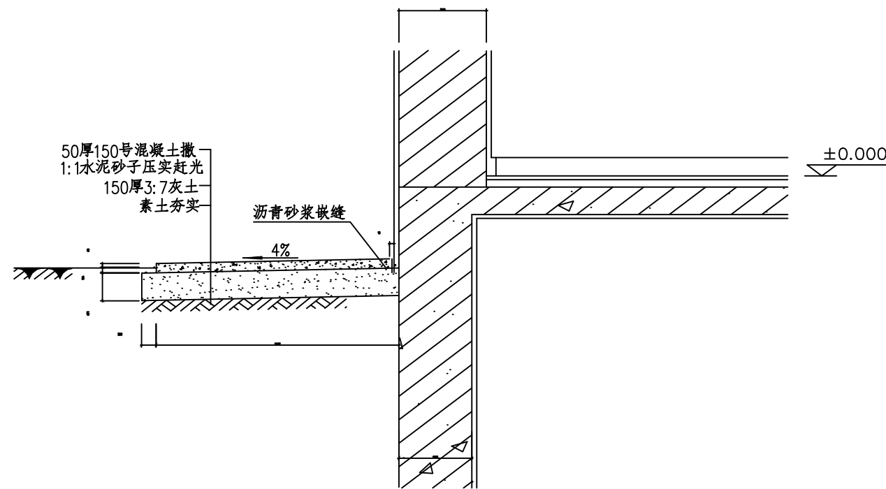
散水大样 1:20
