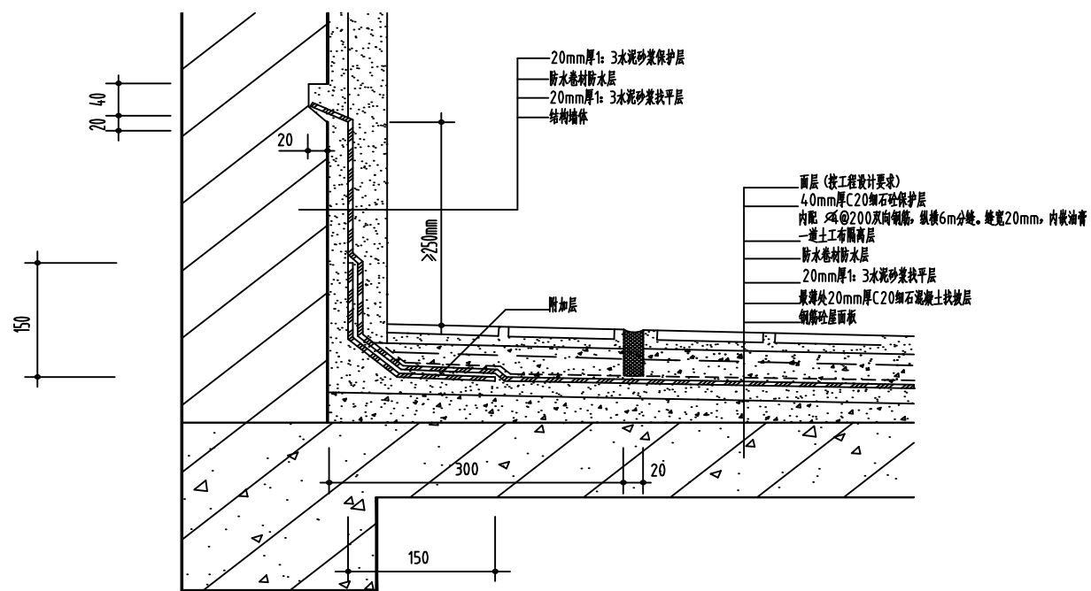
屋面女儿墙防水节点大样1:20
