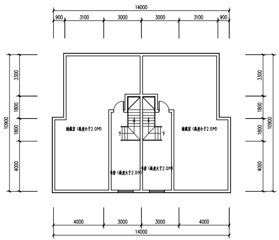
房屋平面图
