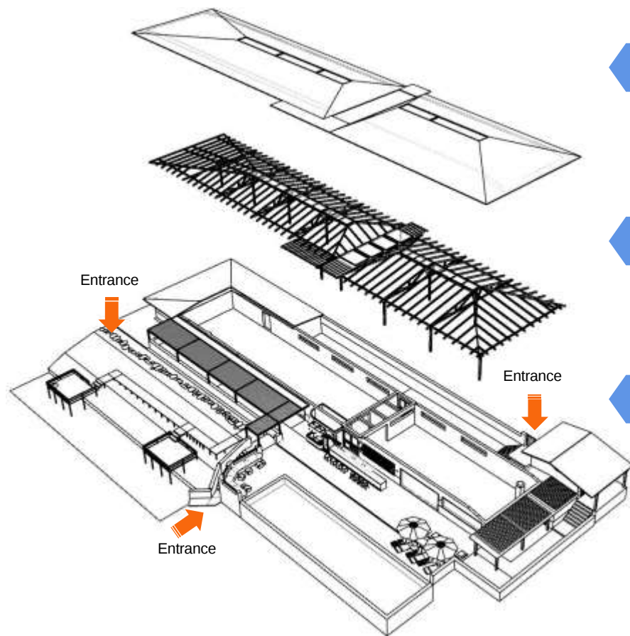
屋面
