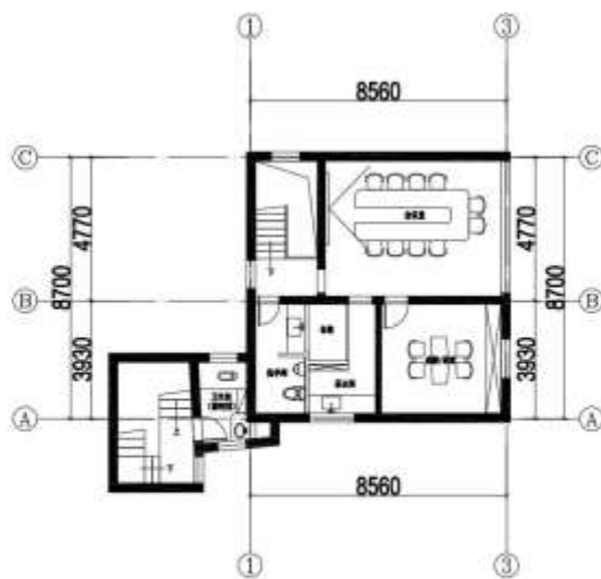
L-2-2F平面布局79m²
