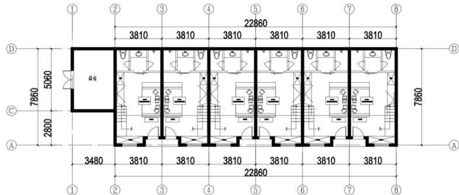
L-5-1F平面布局201m²
