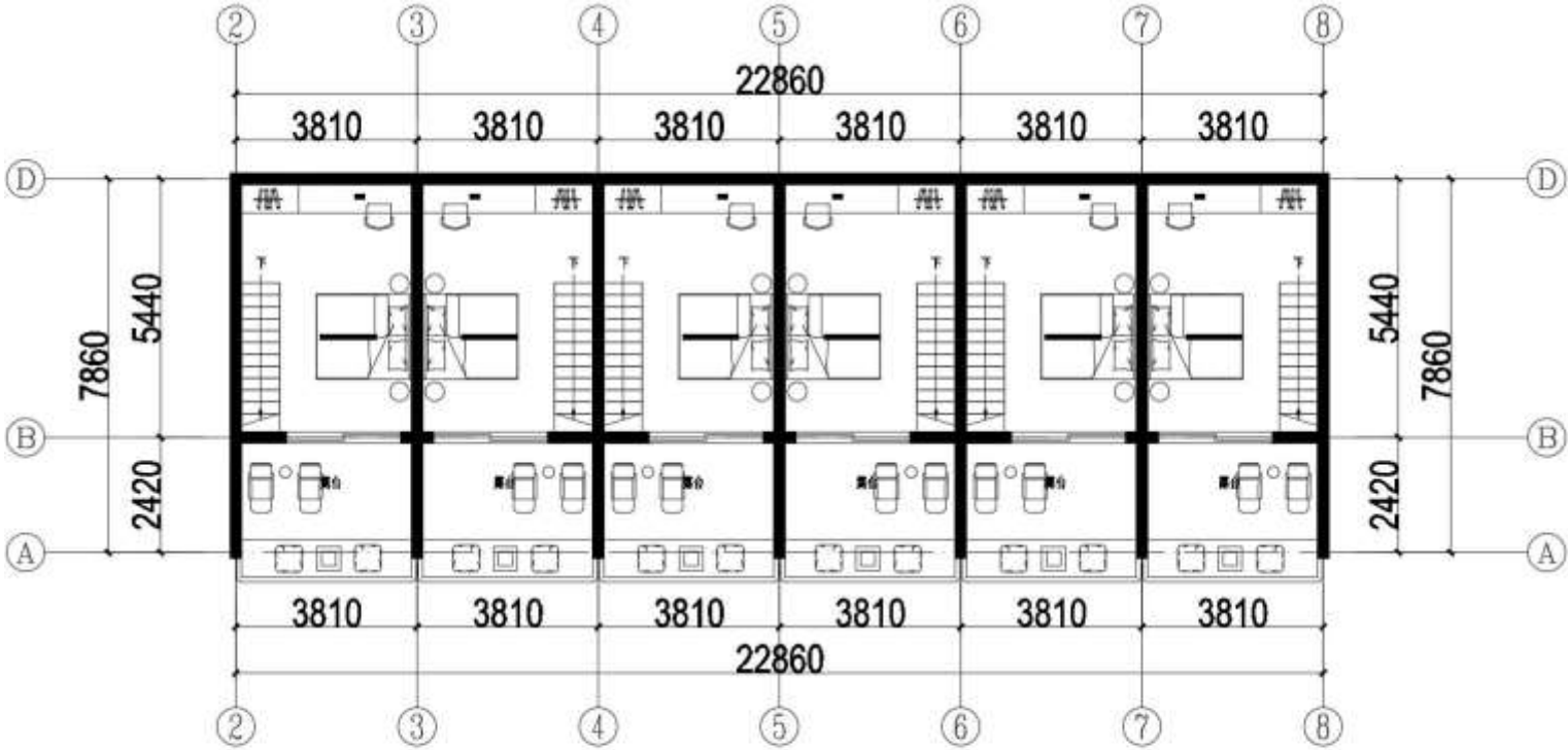
L-5-2F平面布局183m²
