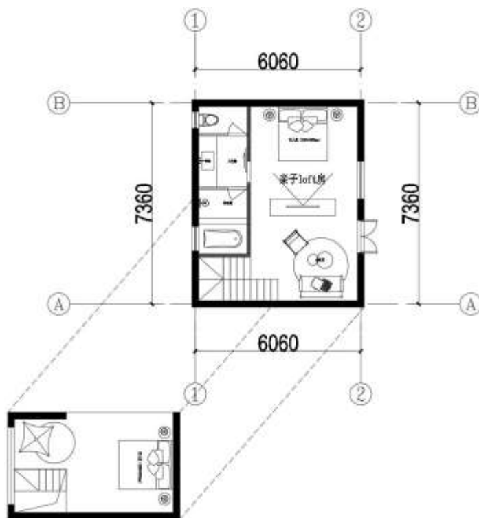
L-3平面布局48m²
