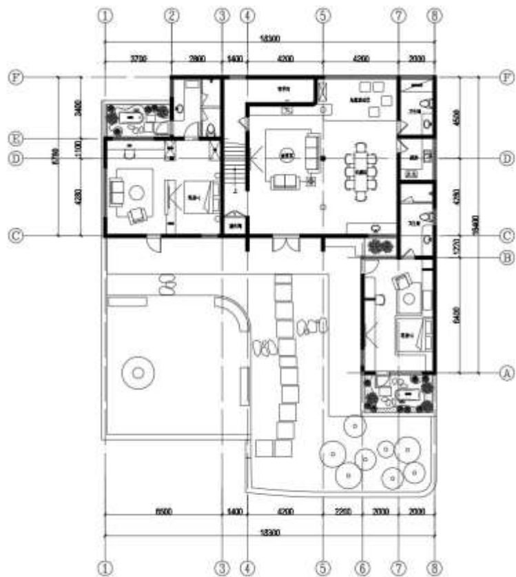
L-9-1F平面布局184m²
