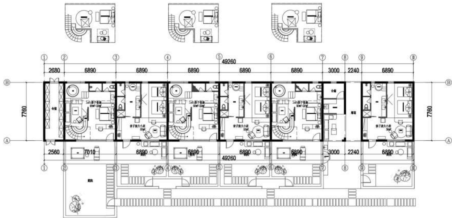
L-7平面布局396m²
